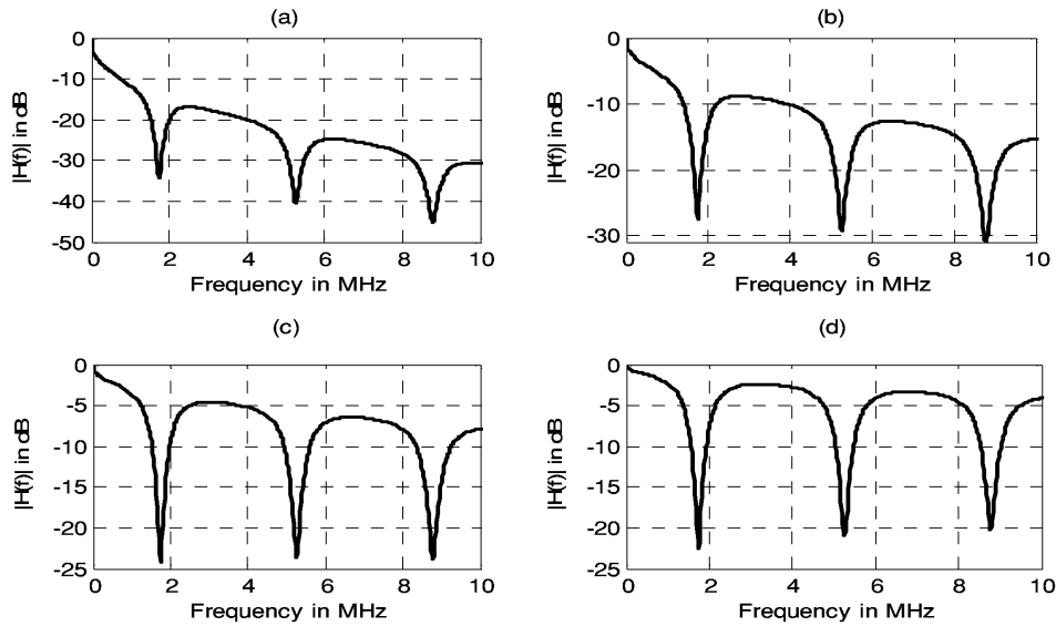
Obr. 6.7: Vliv odbočky na přenosovou funkci pro různé vzdálenosti mezi Tx a Rx: (a) 1,2 km, (b) 600 m, (c) 300 m, (d) 150 m [2].
