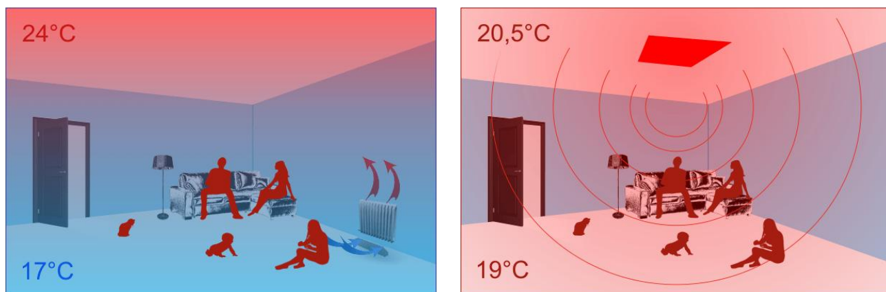
Obr.13 - Princíp vykurovania infranelmi [23]
