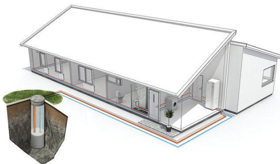
Obr. 6 - Hlbinný vrt [11]
