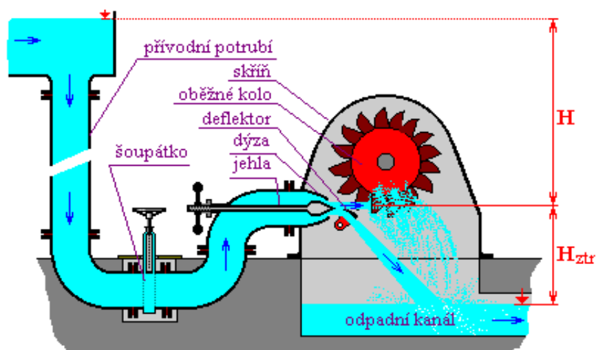
Obr. 7: Peltonova turbína (Zdroj: http://mve.energetika.cz )
