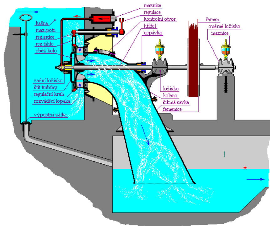
Obr. 5: Francisova turbína (Zdroj: http://mve.energeika.cz )
