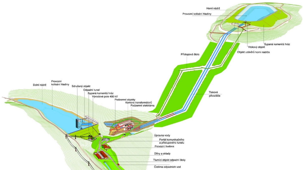
Obr. 15: Znáznornění objektů PVE Dlouhé Stráně (Zdroj: ČEZ).
