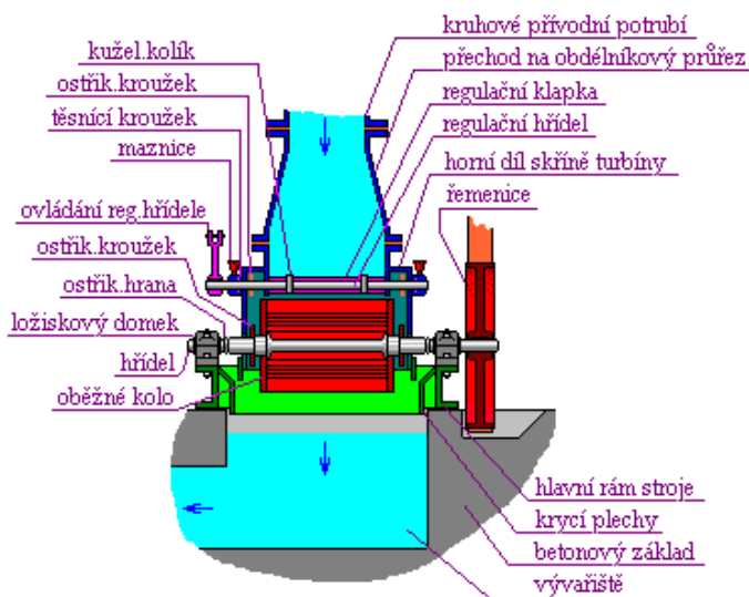
Obr. 8: Bánkiho turbína (Zdroj: http://mve.energetika.cz )
