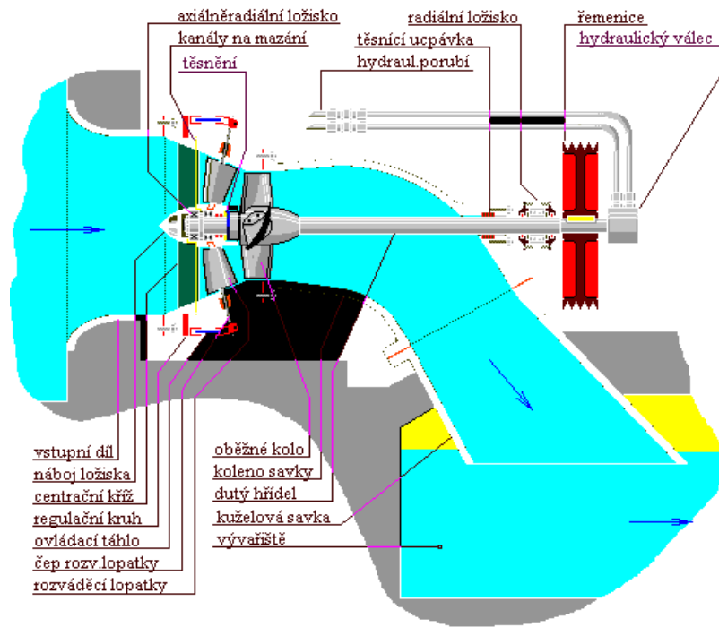
Obr. 6: Kaplanova turbína (Zdroj: http://mve.energeika.cz )
