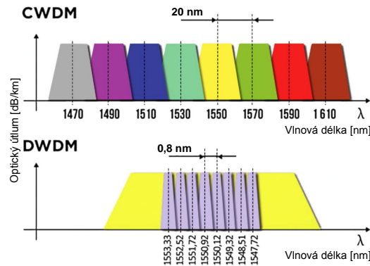
Obr. 4.13: Srovnání CWDM vs DWDM v optickém spektru [40, 41].
