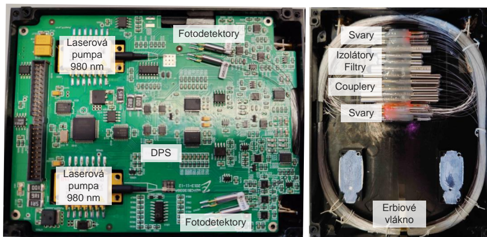
Obr. 2.2: Provedení modulu EDFA zesilovače obsahující booster a preamp.
