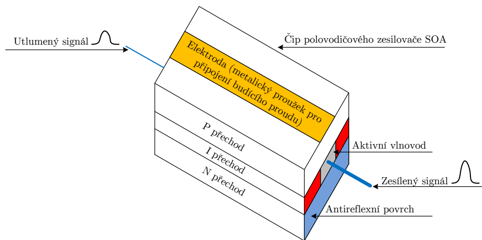
Obr. 2.3: Struktura polovodičového optického zesilovače [3].
