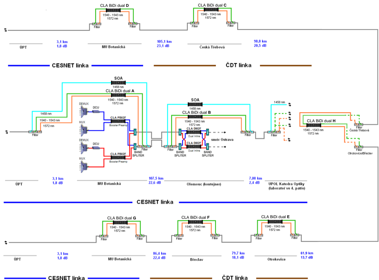
Obr. 4.25: Schéma multiband polygonu pro přenos ultra-stabilních veličin [32, 52].
