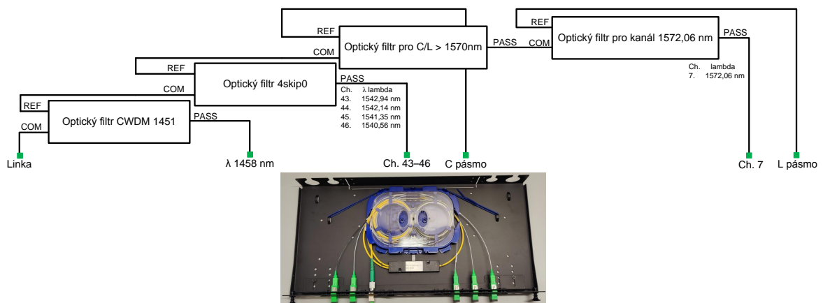
Obr. 4.19: Kompletní provedení zapojení optického filtru pro přenos ultra-stabilních veličin pro multiband polygon pro trasu mezi Brnem a Olomoucí [32].
