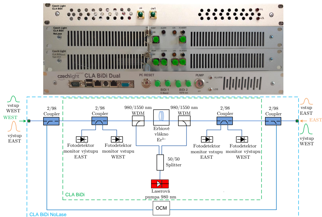
Obr. 4.2: Prototypy CLA BiDi a blokové schéma optické části [2, 12].
