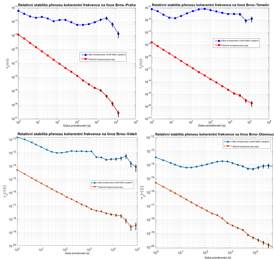
Obr. 4.9: Relativní stabilita přenosu ultra-stabilní frekvence na významných linek v infrastruktuře pro přenos ultra-stabilních veličin [25, 26, 29, 27, 28, 30].
