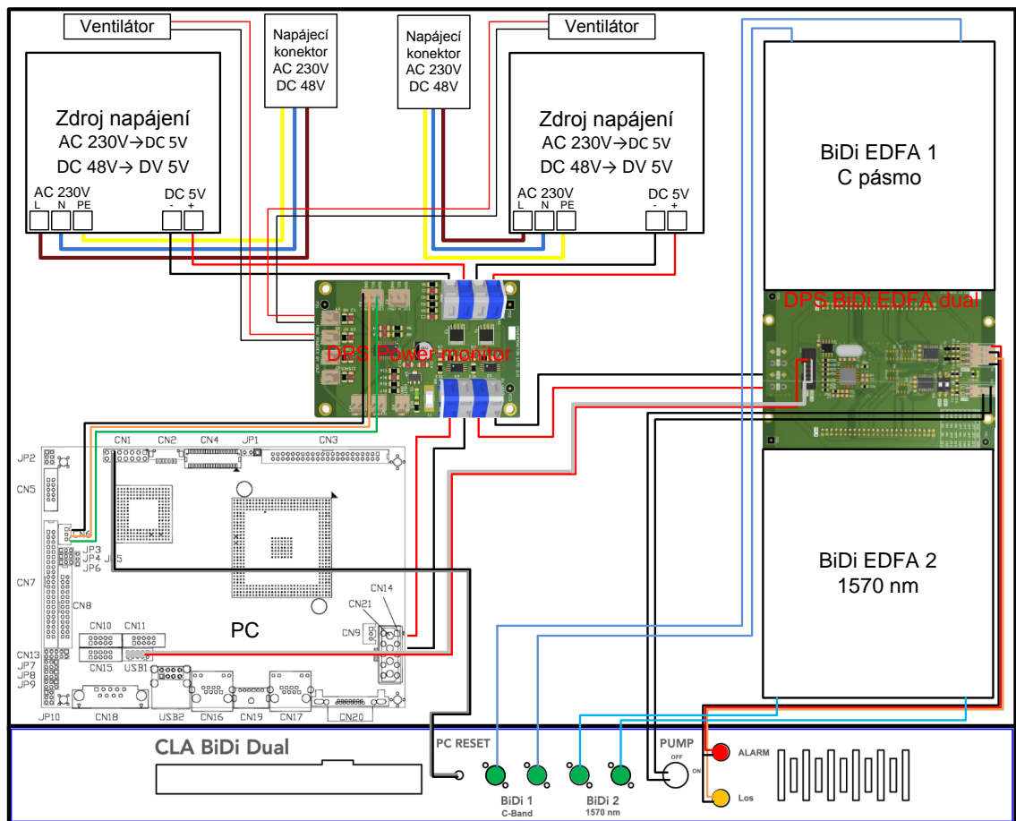
Obr. 4.6: Blokové schéma hardwaru CLA BiDi dual včetně propojů [12].
