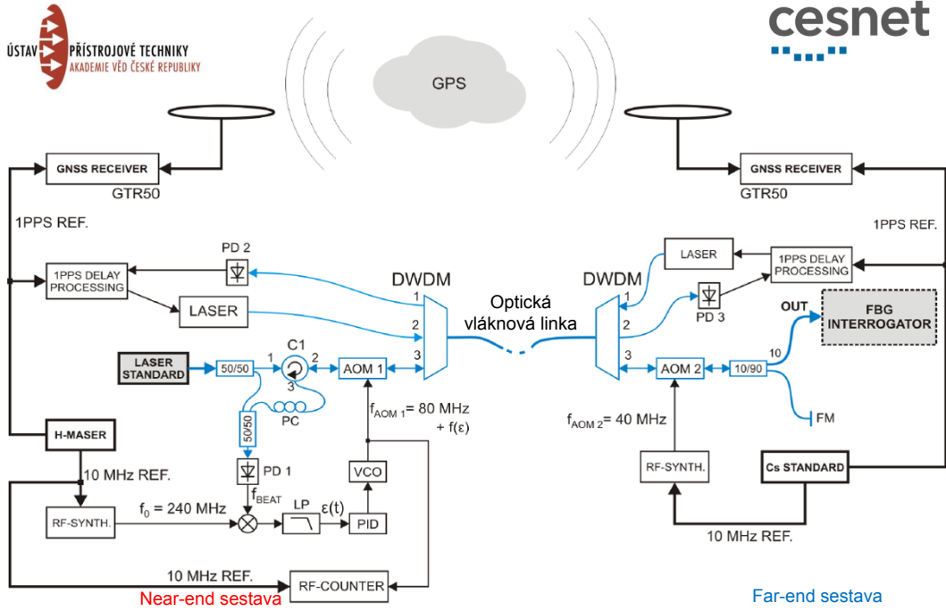
Obr. 4.11: Princip přenosu ultrastabilních veličin [23, 24, 25, 26, 28].
