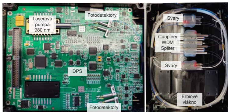
Obr. 4.3: Provedení modulu BiDi EDFA zesilovače.
