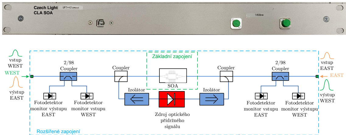
Obr. 4.7: Blokové schéma optické části CLA SOA [10, 11, 13].
