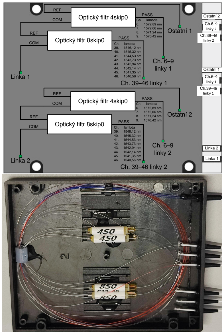
Obr. 4.17: Integrace čtyř optických filtrů do jednoho boxu.
