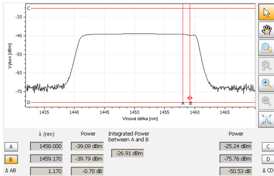
Obr. 4.18: Ověření optického spektra CWDM filtru 1451 pro vlnovou délku 1458 nm.
