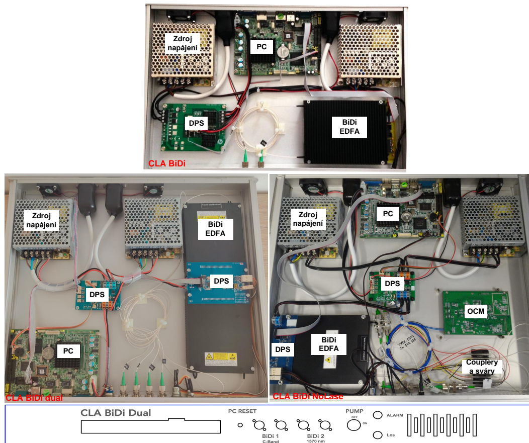
Obr. 4.5: Vývoj vnitřního uspořádání komponent všech prototypů CLA BiDi [2, 12].
