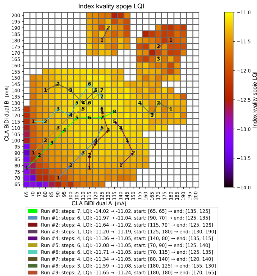
Obr. 4.30: Kombinované výsledky z 10 vyvažovacích běhů vycházejících z 10 různých počátečních stavů pro dva CLA BiDi dual A a B [55].
