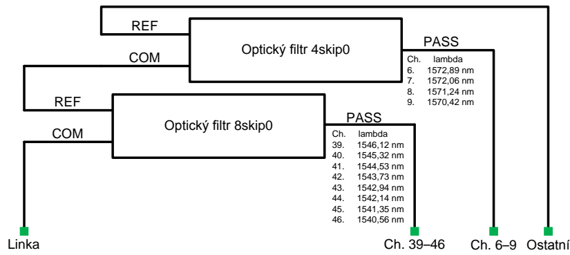
Obr. 4.15: Základní konfigurace zapojení optického filtru pro přenos ultra-stabilních veličin [33].
