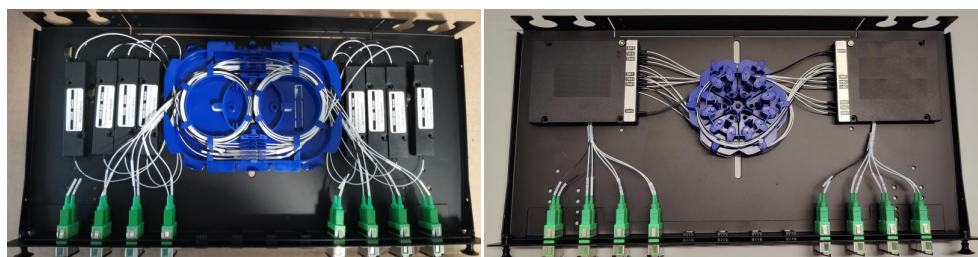
Obr. 4.16: Varianty kompletního provedení zapojení optického filtru pro přenos ultra-stabilních veličin pro překlenutí inline uzlu párové trasy.
