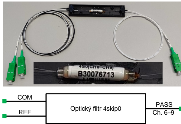
Obr. 4.14: Základní provedení optického filtru.
