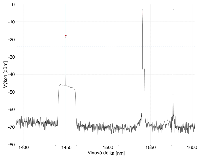
Obr. 4.20: Ověření propustnosti zapojení optického filtru pro přenos ultra-stabilních veličin pro multiband polygon pro trasu mezi Brnem a Olomoucí.
