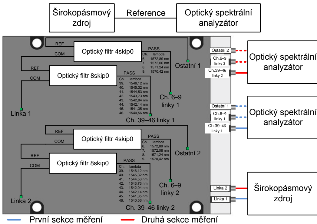
Obr. 4.21: Blokové schéma jednotlivých měření propustnosti optického filtru.
