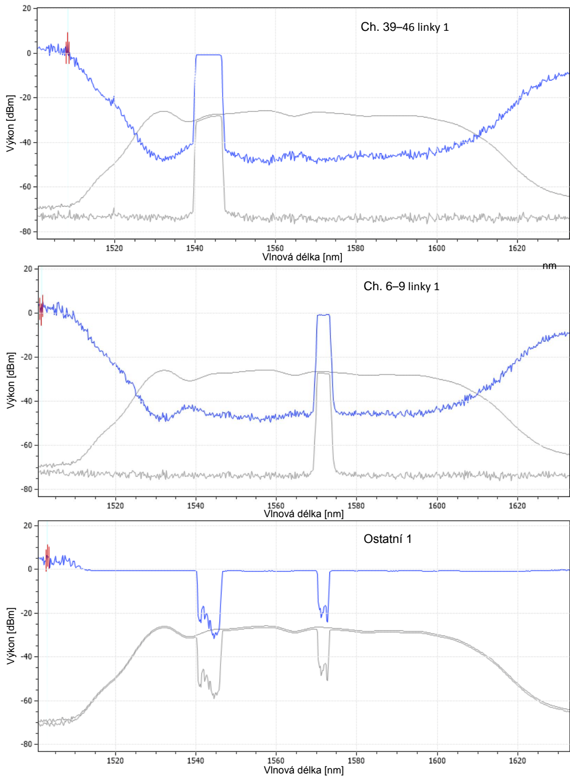
Obr. 4.22: Grafické znázornění propustnosti a strmosti optického spektra na jednotlivých portech modulu, první sekce měření.
