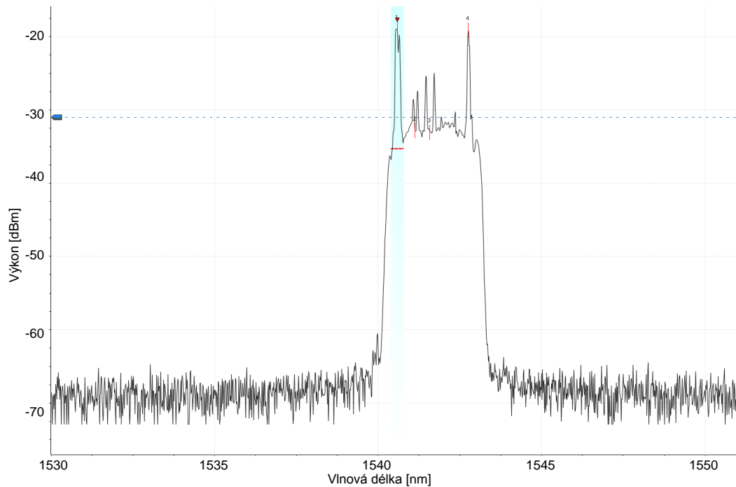
Obr. 4.4: Nežádoucí efekt samovolné laserování (malé peaky uprostřed) [2, 14].
