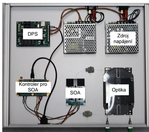
Obr. 4.8: Prototypu CLA SOA základní konfigurace optické části [10, 11, 13].
