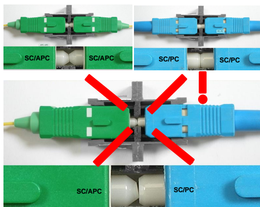
Obr. 4.24: SC konektorové spoje typu APC a PC [50].
