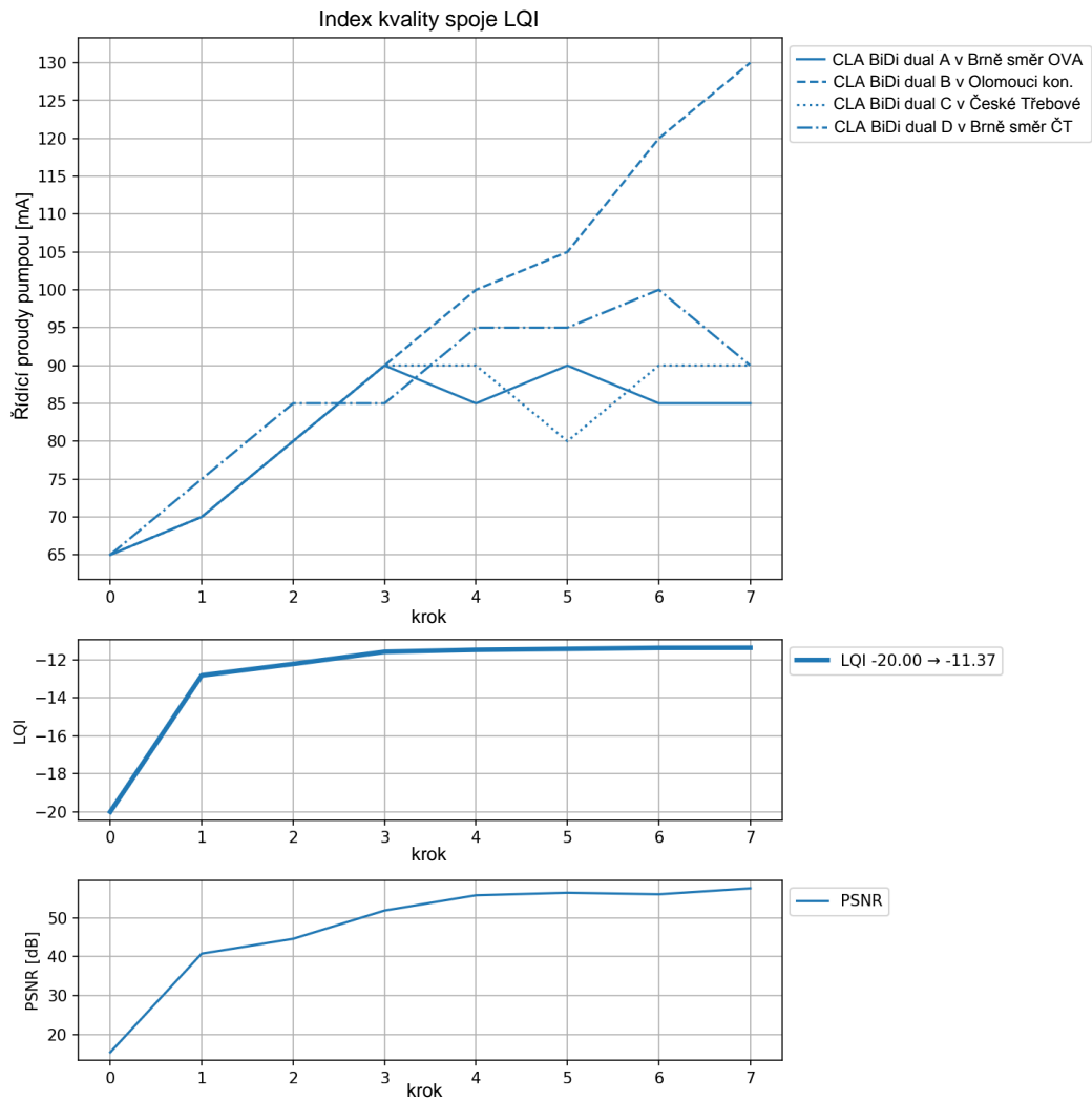
Obr. 4.31: Průběh vyvažovacího běhu č.1 v druhém scénáři pro všechny čtyři obousměrné optické zesilovače CLA BiDi dual [55].
