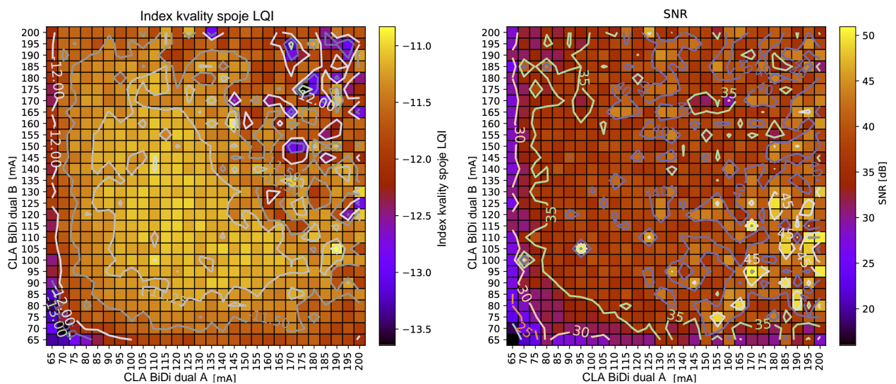
Obr. 4.29: Analýza LQI a SNR před prvními vyvažovacími experimenty [55].
