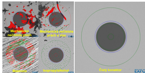
Obr. 4.23: Ukázka špinavého a čistého konektoru.
