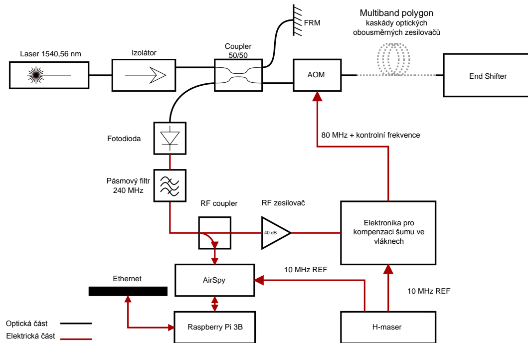
Obr. 4.28: Blokové schéma experimentálního uspořádání s Michelsonovým interferometrem sloužící k určení LQI [30, 55].
