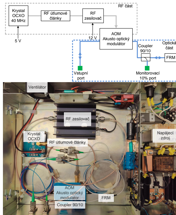
Obr. 4.12: Blokové schéma a provedení prototypu end-shifteru.
