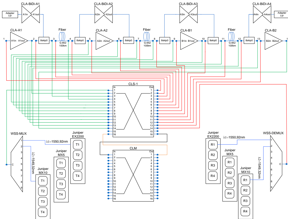
Obr. 4.1: Blokové zapojení současného dynamického testbedu.
