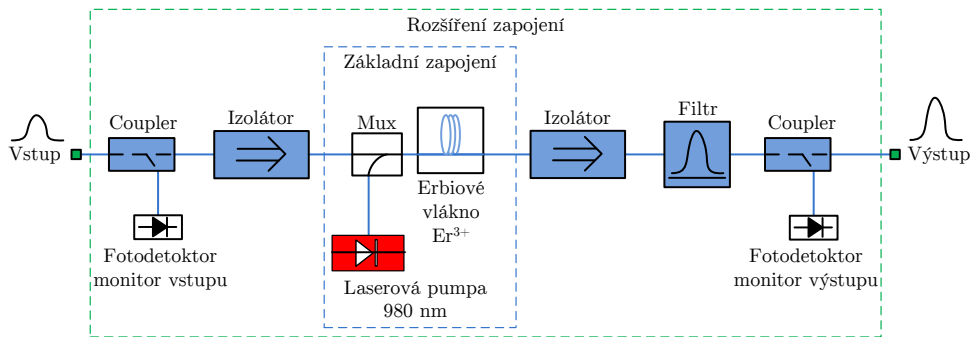
Obr. 2.1: Blokové zapojení vláknového zesilovače EDFA [2].
