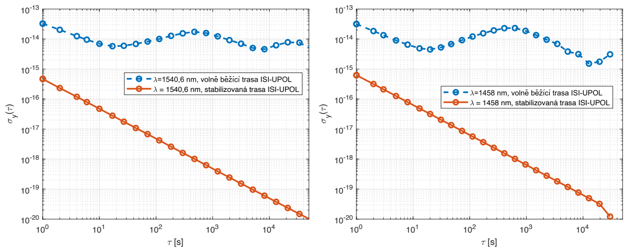
Obr. 4.27: Měřená stabilita linek přenosu ultra-stabilní frekvence metodou in-loop v multiband polygonu.
