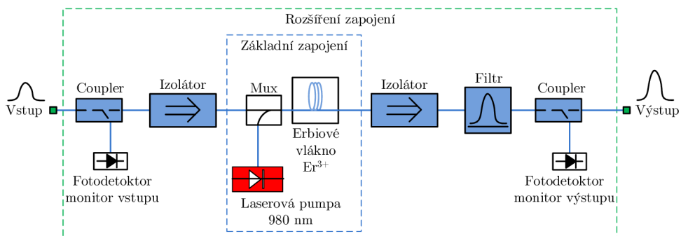
Obr. 2.1: Blokové zapojení vláknového zesilovače EDFA [2].
