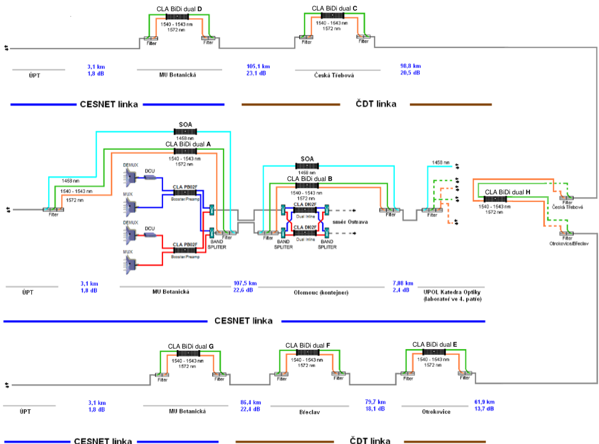
Obr. 4.25: Schéma multiband polygonu pro přenos ultra-stabilních veličin [32, 52].
