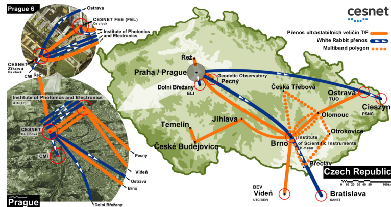
Obr. 4.10: CESNET infrastruktura pro přenos ultra-stabilních veličin [2, 23, 24, 33, 34].
