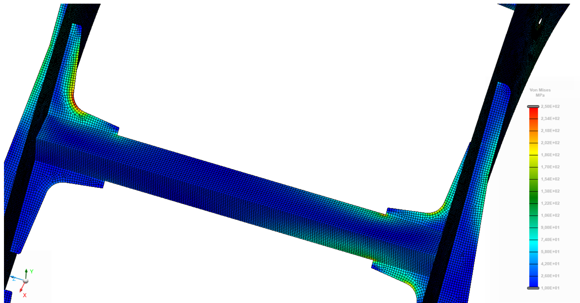
Příloha IV: Detail koncentrace napětí ve výstužných žebrech při průjezdu zatáčkou, rozsah zobrazení napětí (0-285 MPa)
