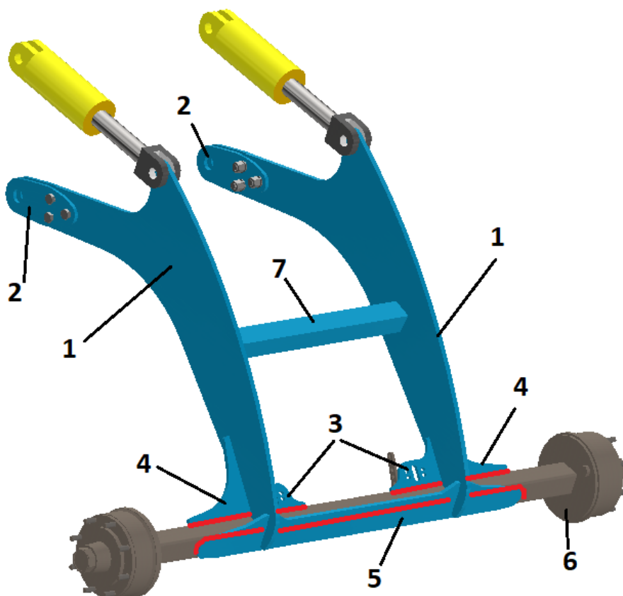
Obrázek 19: Prvotní návrh svařence nápravy, 1 – hlavní nosné plechy, 2 – připojovací bočnice, 3 – vnitřní výstuha, 4 – vnější výstuha, 5 – zadní pásnice, 6 – nakupovaná náprava, 7 – příčný nosník čtvercového profilu
