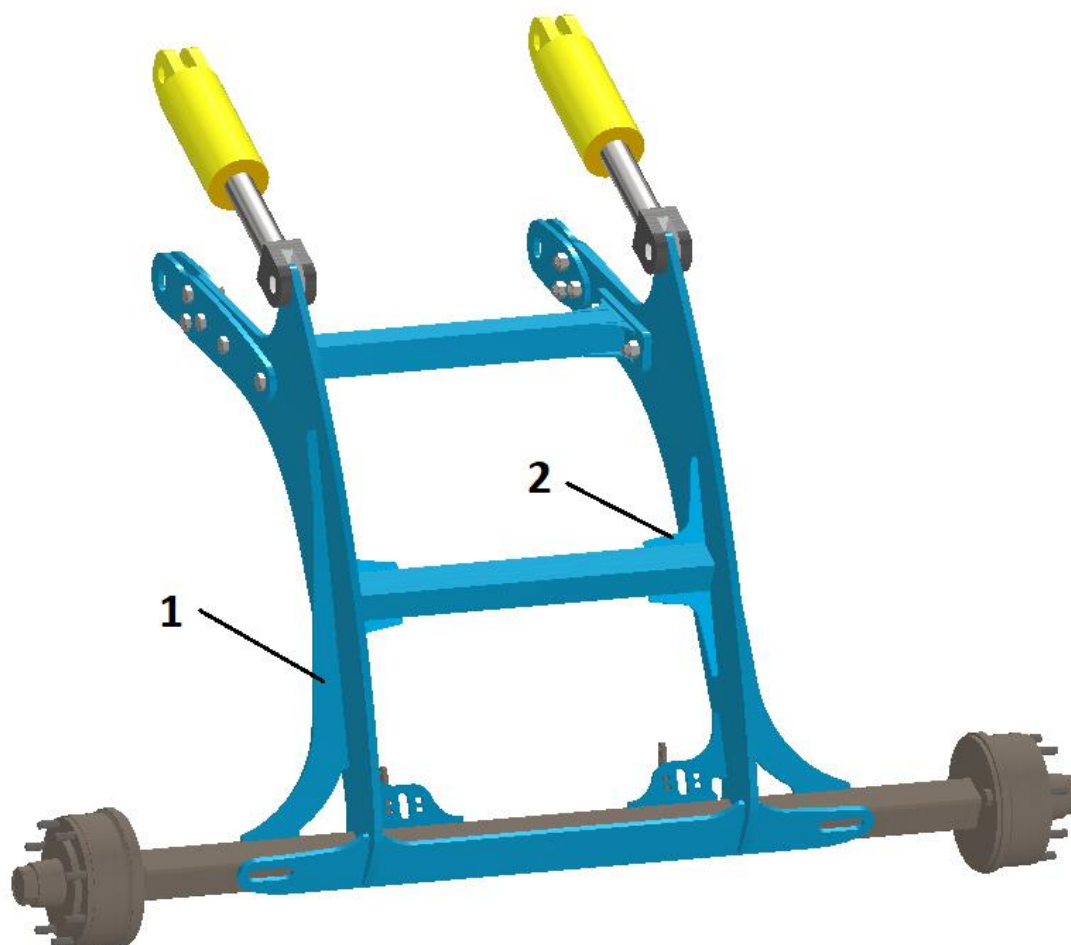
Obrázek 35: Druhá verze úprav nápravy, 1 – prodloužený tvar vnějších výztužných žeber, 2 – přidaná žebra pro ochranu svaru nosných plechů a příčného profilu
