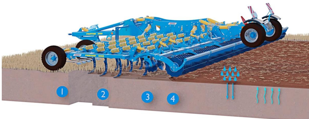
Obrázek 1: Dlátový kypřič Fantom CLASSIC, 1 – flexi-cut pro urovnání před přípravou, 2 – šípovité radličky pro mělkou podmítku půdy, 3 – zahrnovací disky, 4 – zavlačovací válce [5]
