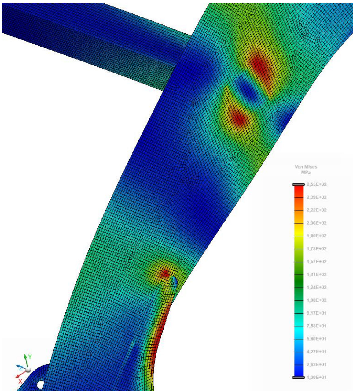
Obrázek 25: Detail koncentrace napětí v místě svaření příčného čtvercového profilu a vnějšího výtuzného žebra s nosným plechem prvotního návrhu konstrukce při průjezdu zatáčkou, rozsah zobrazení napětí (0–255 MPa)
