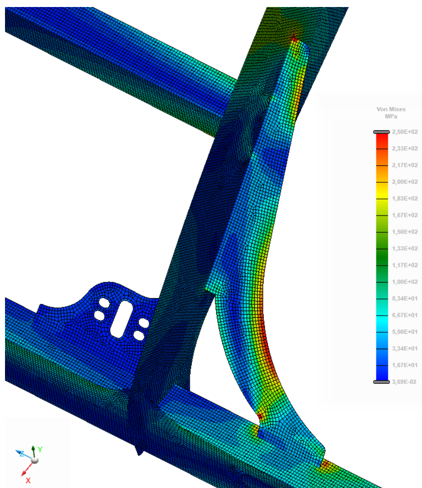
Obrázek 32: Zobrazení napětí na vnějším výztužném žebro upravené konstrukce nápravy pro zatěžování při průjezdu zatáčkou, rozsah zobrazení napětí (0-250 MPa), škála stupnice byla upravena, aby byla zřetelněji viditelná místa s nebezpečným napětím ve svarových spojích konstrukce
