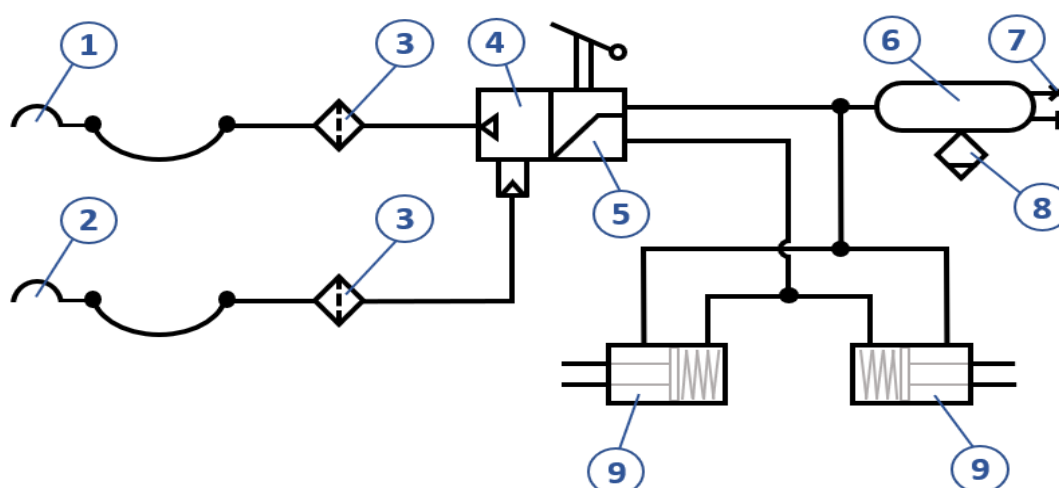
Obrázek 12: Schéma dvouhadicové vzduchové soustavy
