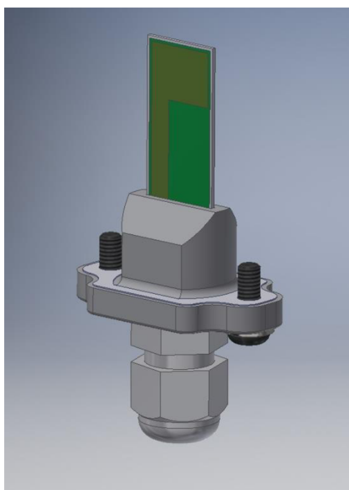
Obrázek 24 – Kompletní jiskřiště k montáži [Vlastní zpracování]
