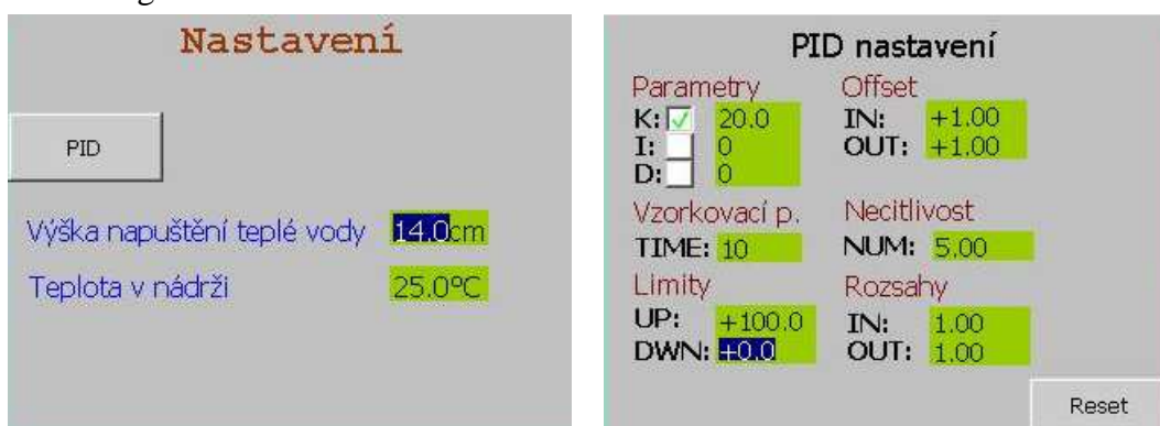
Obrázek 15, obrazovky pro nastavení automatického režimu
