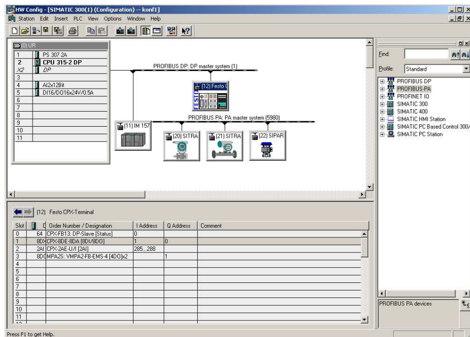
Obrázek 9, nastavení ventilového ostrovu v HW Config
