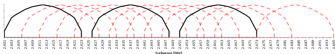
Obr. 1.2: Rozložení kanálů v DSSS
