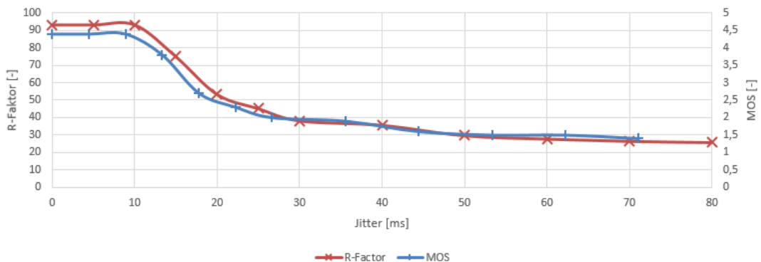
Obr. 6.18: Vliv změny jitteru na MOS/R-Faktor
