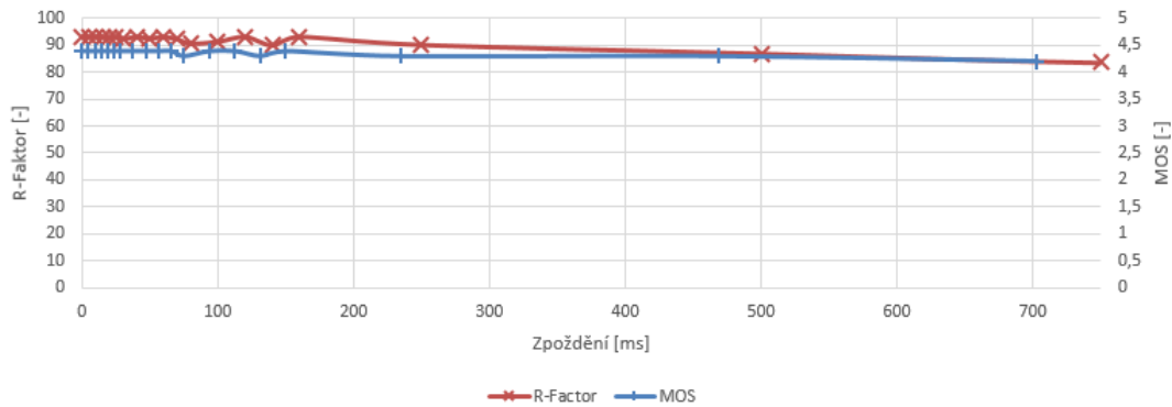
Obr. 6.17: Vliv změny zpoždění na MOS/R-Faktor
