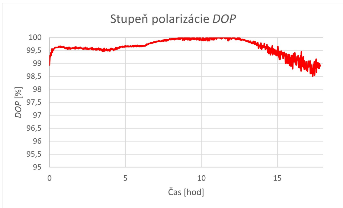
Obr. 4.9: Znáozornenie stupňa polarizácie DOP
