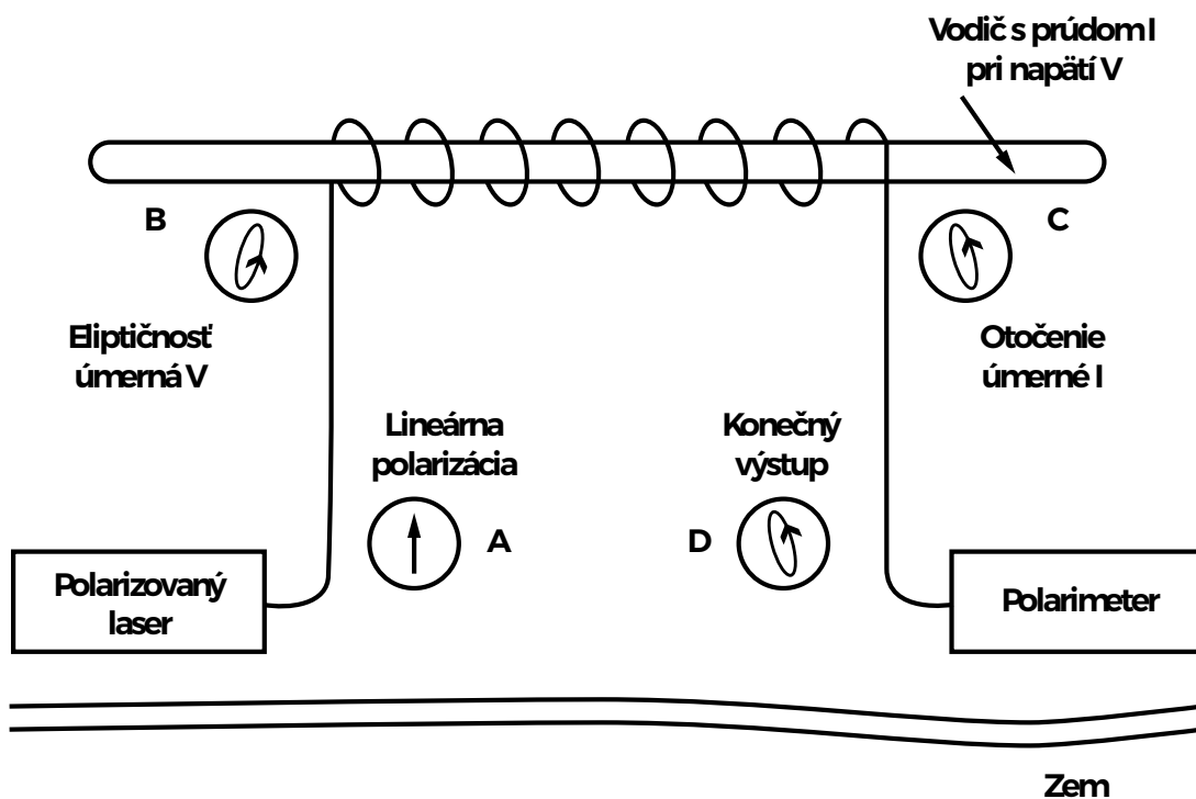
Obr. 1.11: OVS na súčasné meranie prúdu a napätia vo výkonových vedeniach
