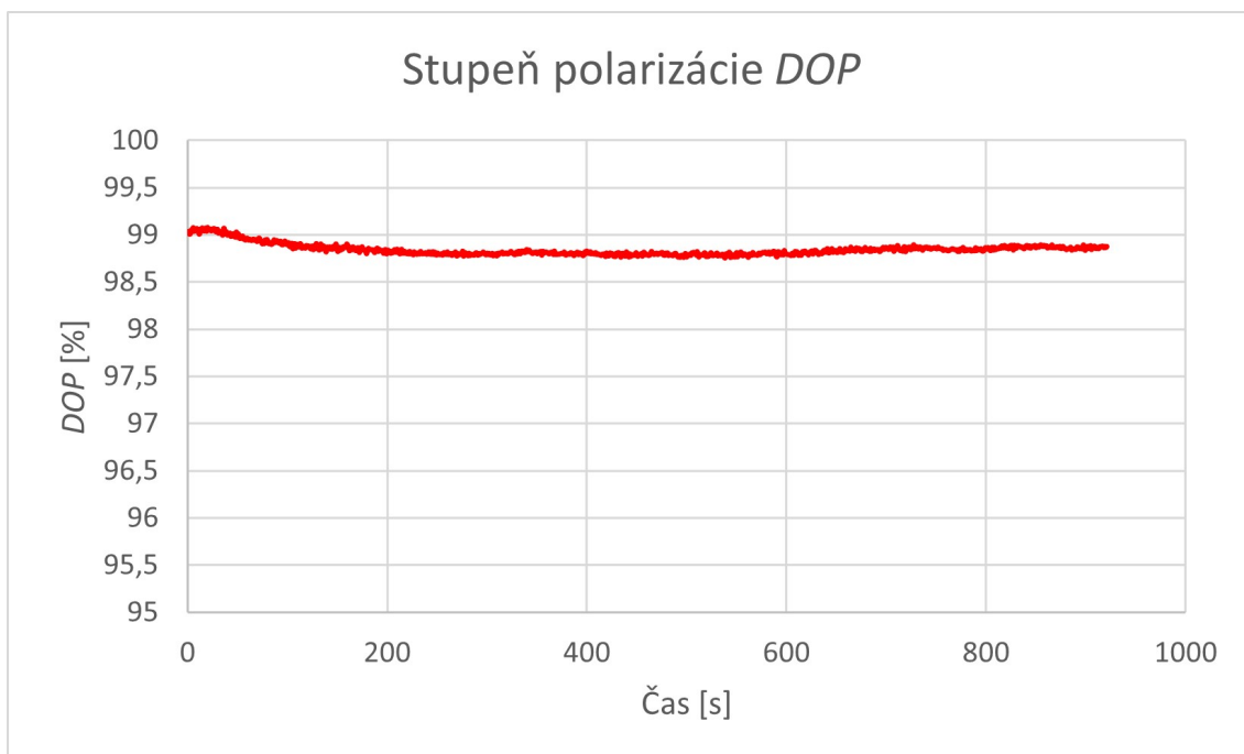
Obr. 4.17: Znázornenie stupňa polarizácie DOP
