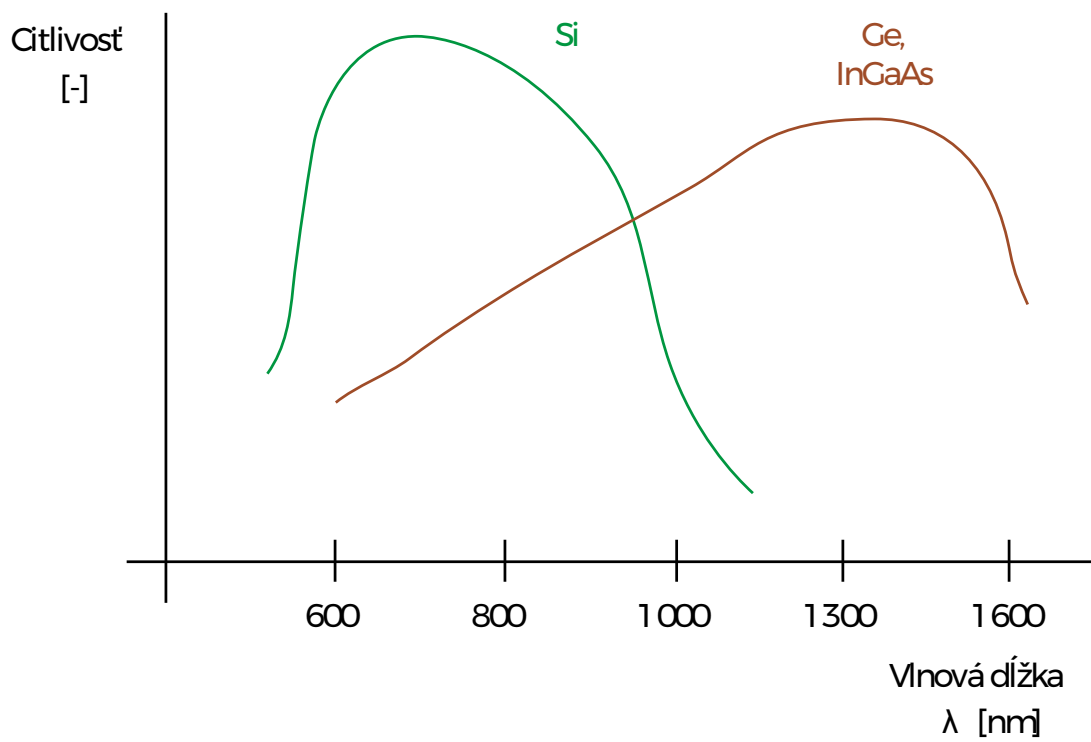
Obr. 2.4: Cítlivost detektorov Si, Ge, InGaAs v závislosti od vlnovej dĺžky a materiálu
