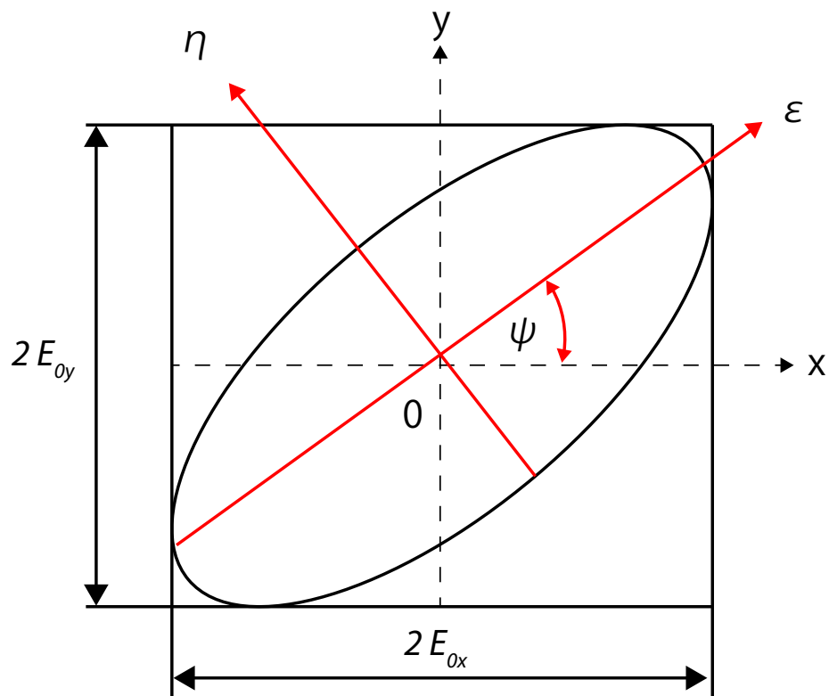
Obr. 1.5: Polarizačná elipsa
