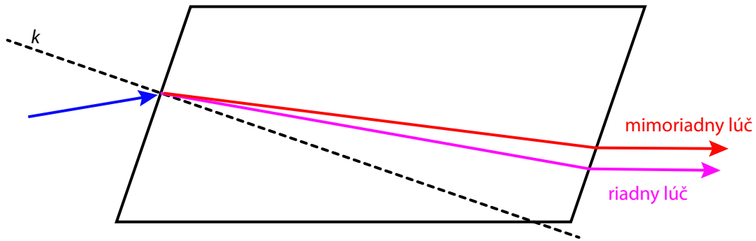
Obr. 1.3: Polarizácia dvojlomom
