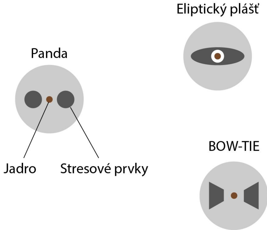
Obr. 1.4: Priečny rez PMF typu PANDA, BOW-TIE a Elipsa
