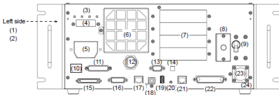
Obrázek 3: Zadní panel řídicí jednotky RC700-A
