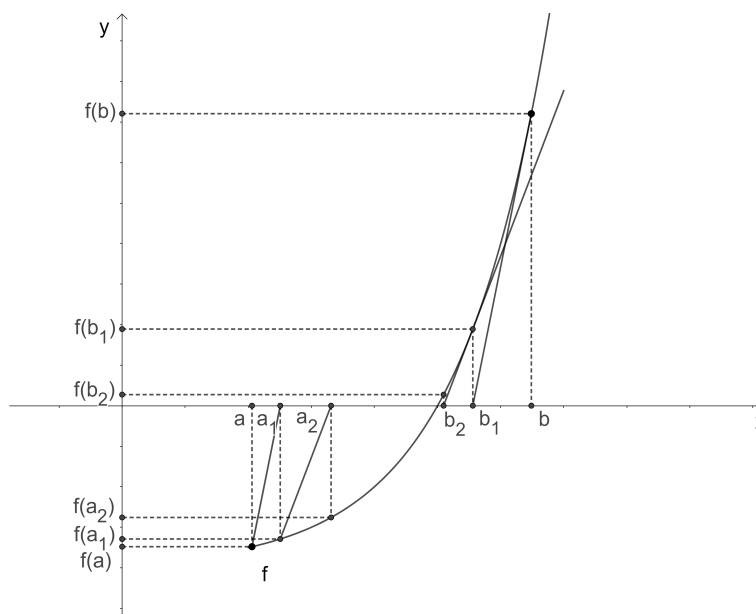
Obrázek 2.2: Newtonova metoda
