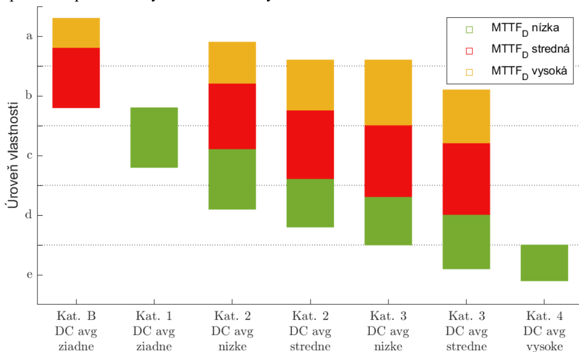
Obrázok 1 Určenie hodnoty PL [1]
