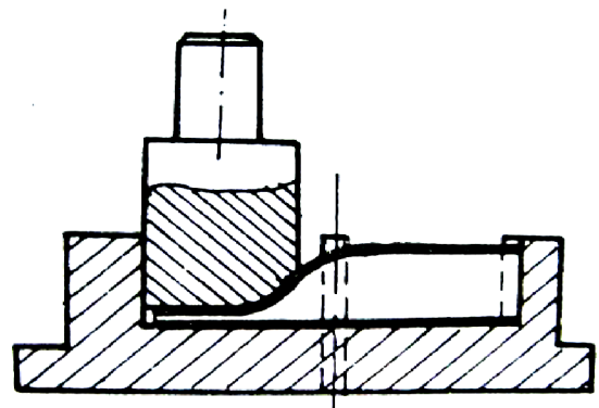
Obr. 15 Přípravek na zplošťování trubek pro nesymetrické zploštění [1]
