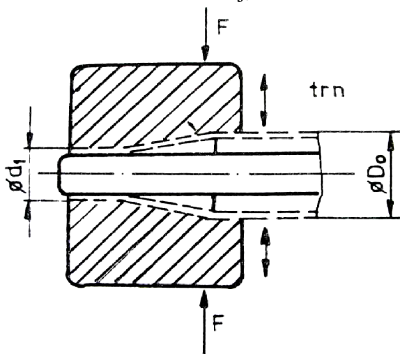
Obr. 14 Zužování trubky s užitím kalibračního trnu [1]
