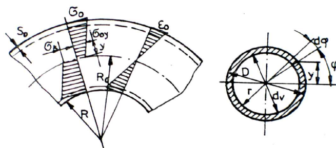
Obr. 20 Rozložení osového napětí a přetvoření [1]
