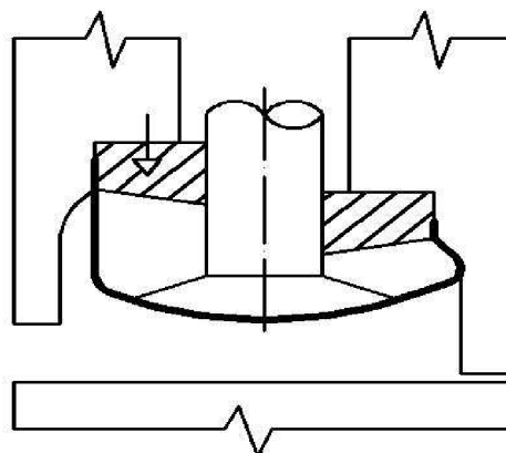
Obr. 9 Radiální vypínání
