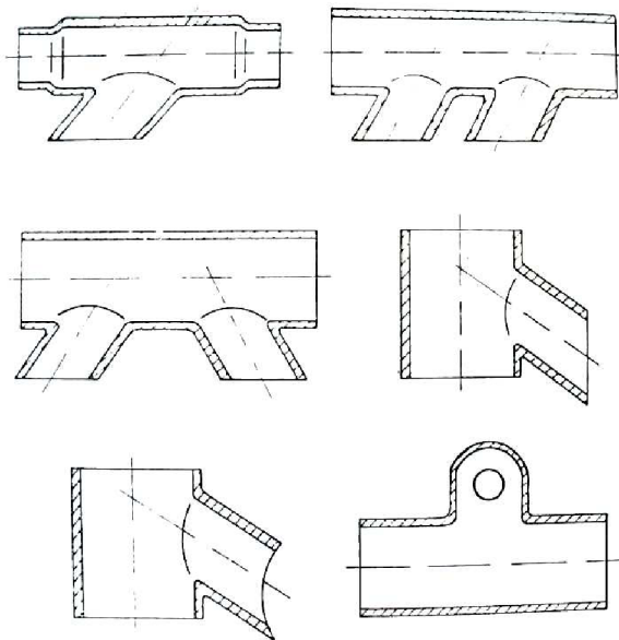
Obr. 6 Asymetrické součásti Součásti potrubí [4]
