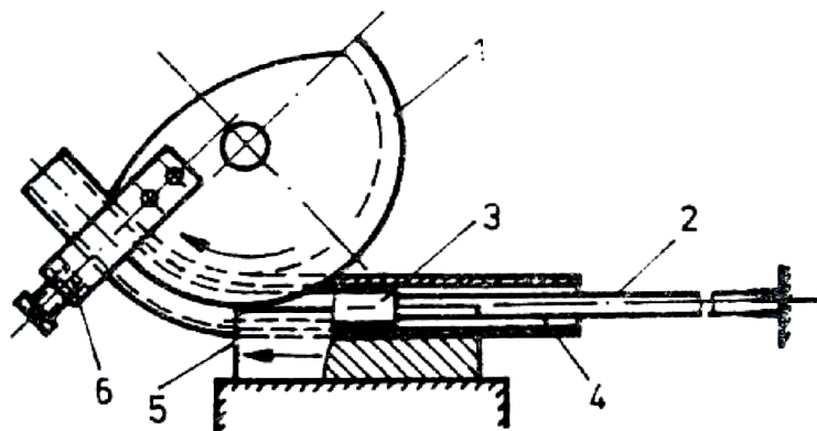
Obr. 29 Ohyb navíjením [1]
