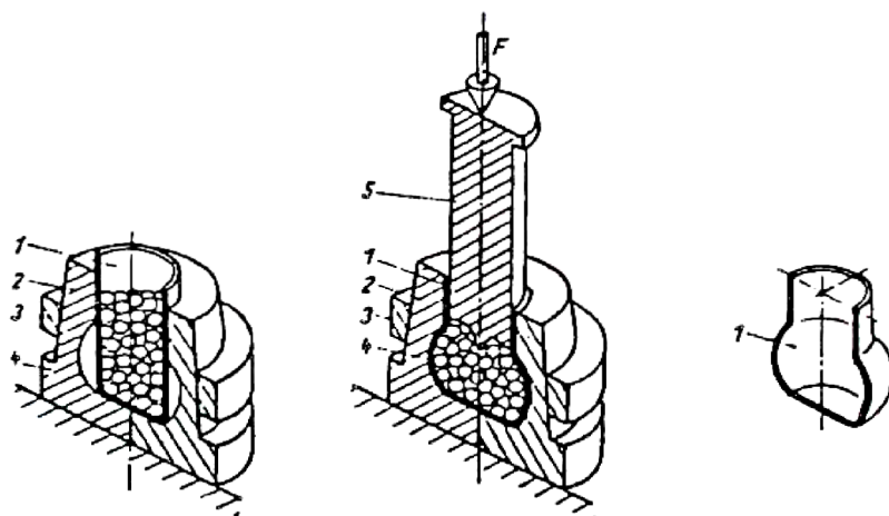
Obr. 26 Výplň pomocí ocelových broků [8]
