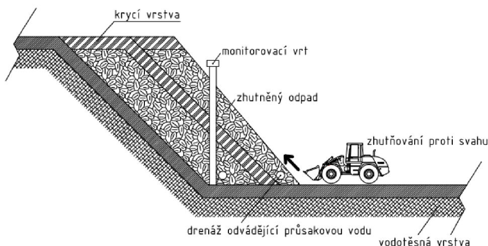
Obr. 11 - Vzorová schémata skládek ve svahu a na rovině [vlastní]
