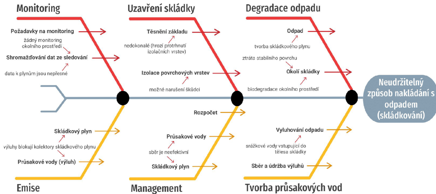
Obr. 16 - Ishikawa Diagram – skládkování [vlastní]
