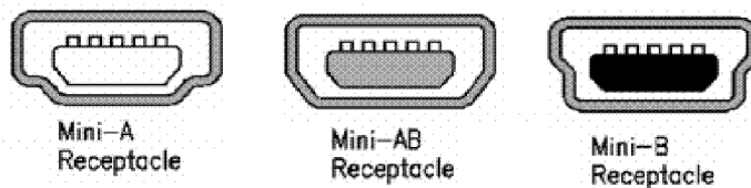
Obrázek 2.9: Mini USB konektory (zleva pro EH, OTG, koncové zařízení).
