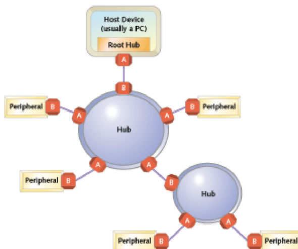
Obrázek 2.6: Topologie sběrnice USB. Obrázek převzat z [7].
