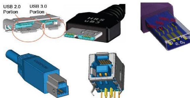
Obrázek 2.8: Konektory standardu USB 3.0. Obrázky převzaty z [9] a [10].
