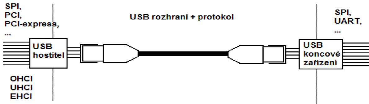
Obrázek 2.7: Znárodnění částí rozhraní.
