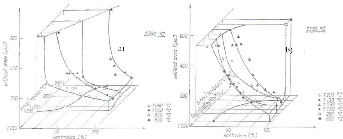
Obr. 2 Rekrystalizační diagramy lité oceli 08Ch18N10T pro počáteční teplotu ohřevu a) 1090 °C, b) 1250 °C.
