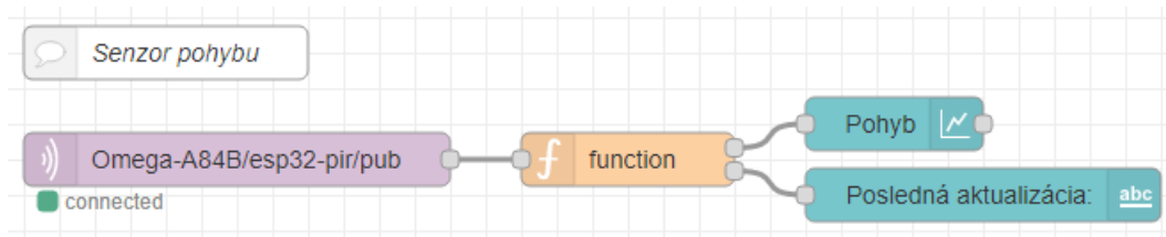
Obr. 5.5: Zobrazenie toku senzora pohybu v Node-RED
