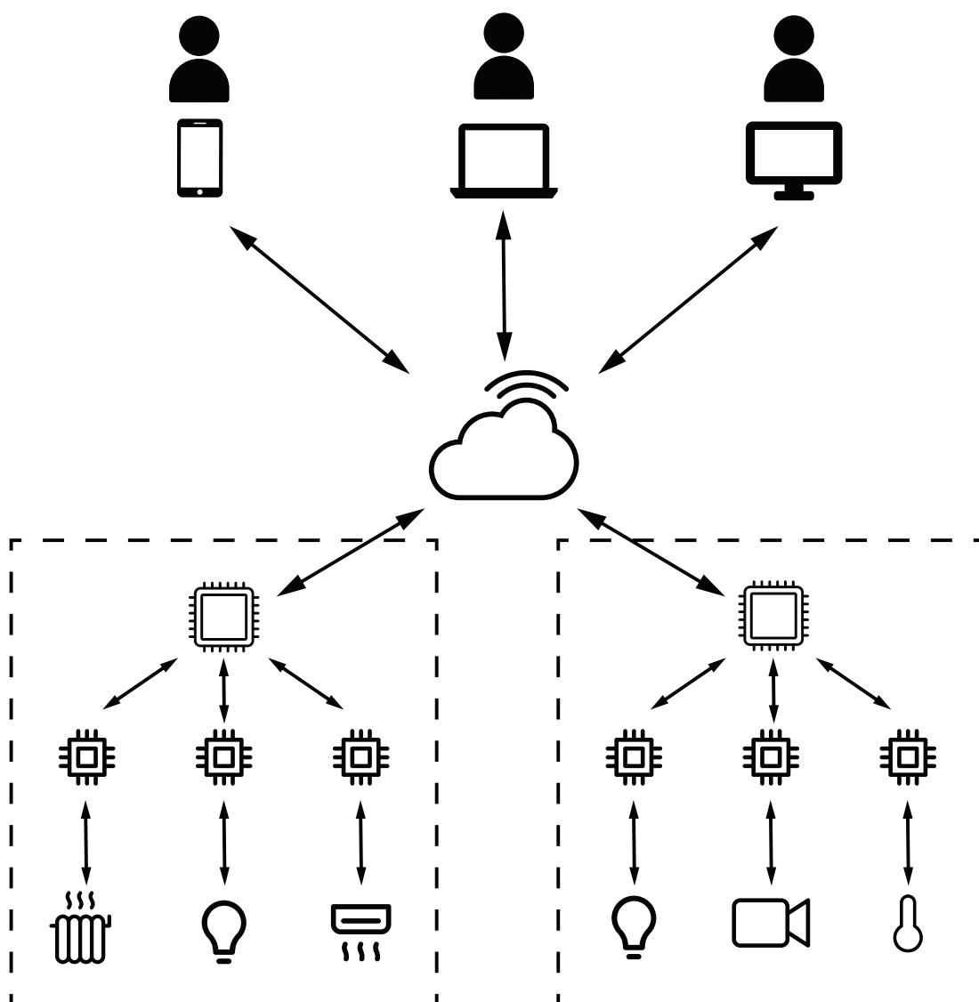
Obr. 4.1: Architektúra systému. Užívatelia sa pomocou zariadení pripájajú na cloud, odkiaľ prebieha monitorovanie a ovládanie systému. Ku cloudu sú pripojené zariadenia Onion Omega2, na ktoré sú ďalej napojené mikrokontroléry so senzormi a aktuátormi. Prerušovanou čiarou sú znázornené oblasti.
