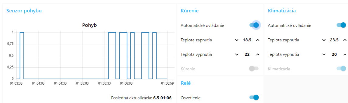
Obr. A.2: Grafické rozhranie monitorovacieho a riadiaceho systému. Časť 2/2
