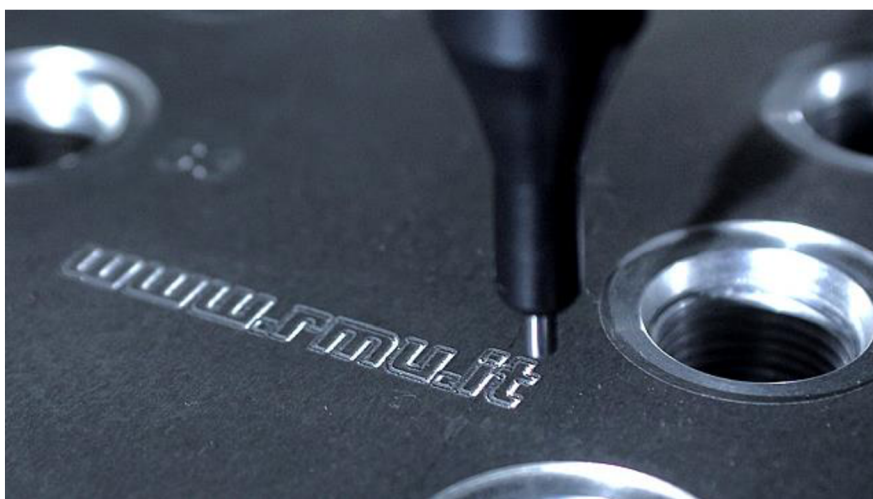
Obrázek 14: Značení rytím [4]
