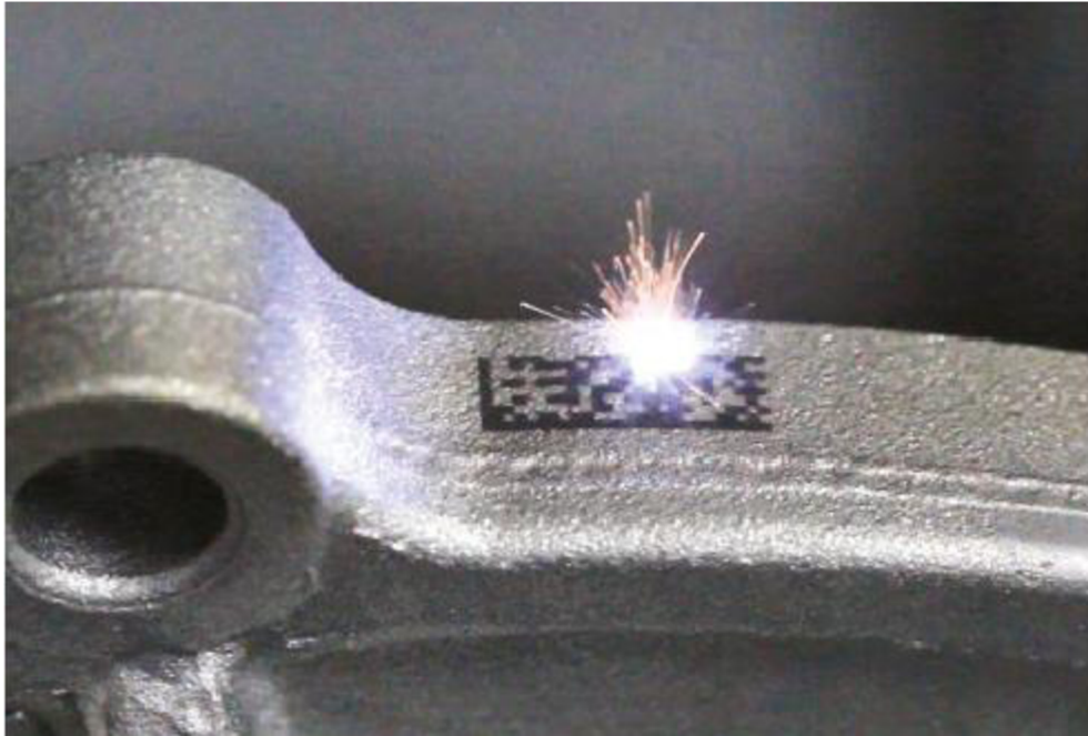
Obrázek 18: Značení DMC kódu na hliníkový odlitek [17]
