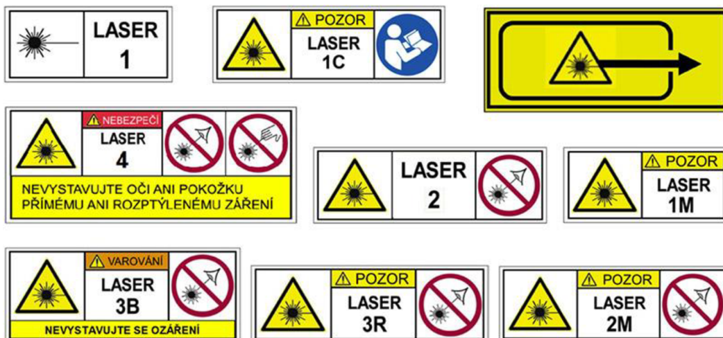
Obrázek 19: Alternativní výstražné štítky pro laserová zařízení [4]
