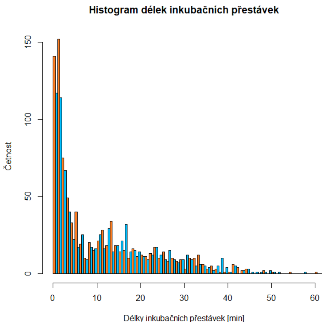
Obrázek 12: Histogram četnosti délek inkubačních přestávek pro jednotlivé druhy. Oranžová barva představuje bekasinu otavní a modrá sluku lesní.
