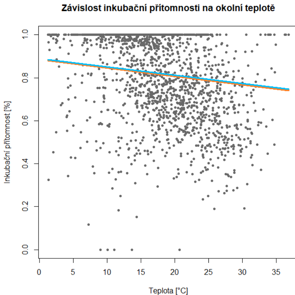
Obrázek 16: Graf závislosti inkubační přítomnosti na okolní teplotě. Osa y představuje inkubační přítomnost jedince na hnízdě. Na ose x jsou teploty okolí udávány ve °C.. Šedé tečky zobrazují nasbíraná data pro inkubační sezení. Modrá linie znázorňuje sluku lesní a oranžová bekasinu otavní. Linie byly vykresleny na základě modelu pro celkovou inkubační přítomnost v průběhu dne v rámci jednotlivých hodin.
