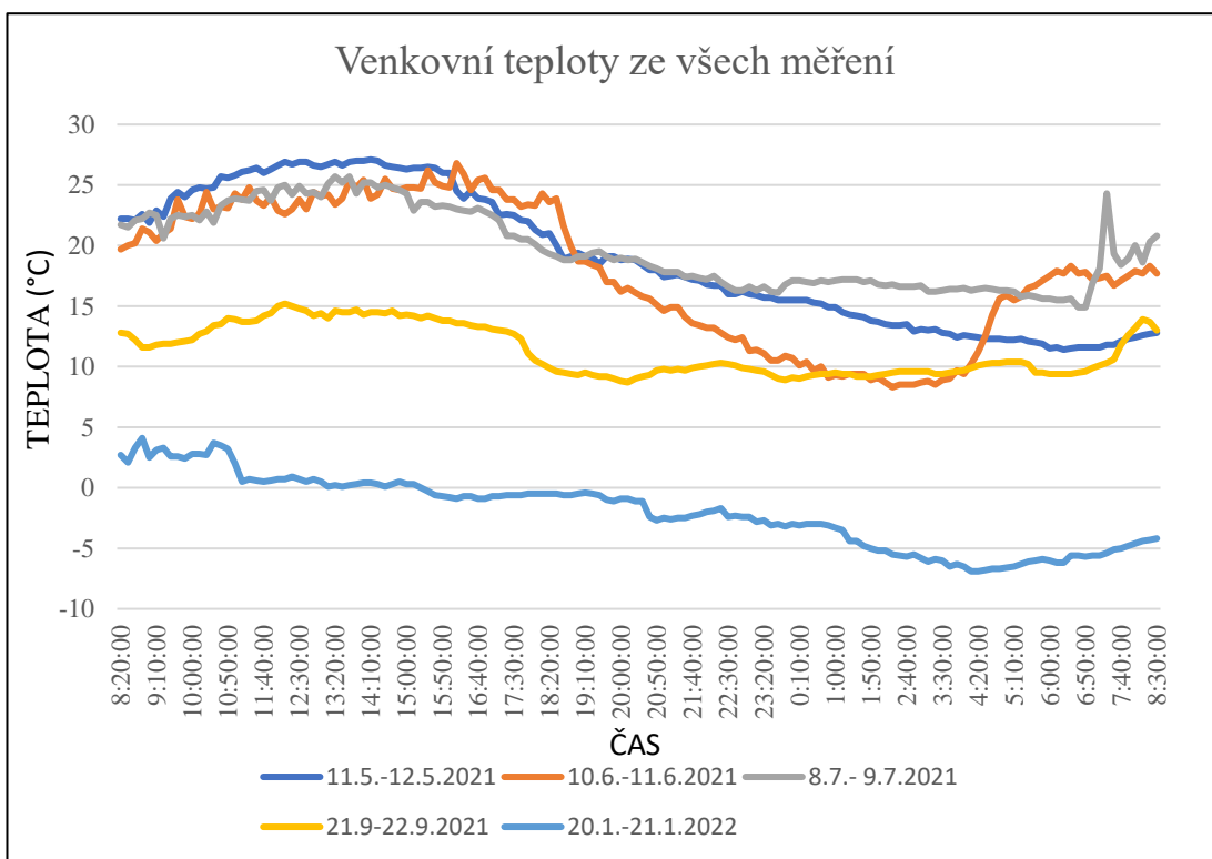
Obrázek 4.6: Venkovní teploty ze všech měření
