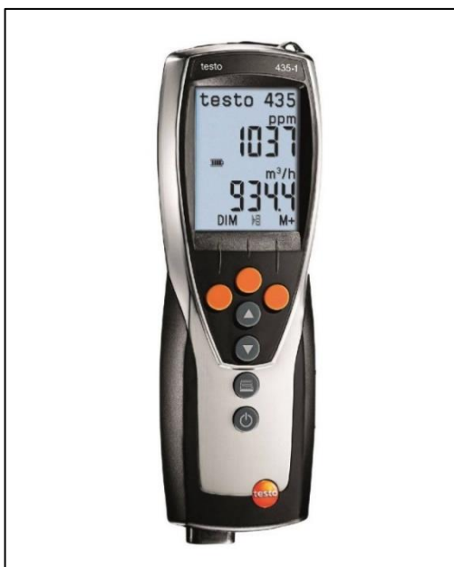
Obrázek 3.4: Anemometr Testo 435 (conrad.cz, 2021)
