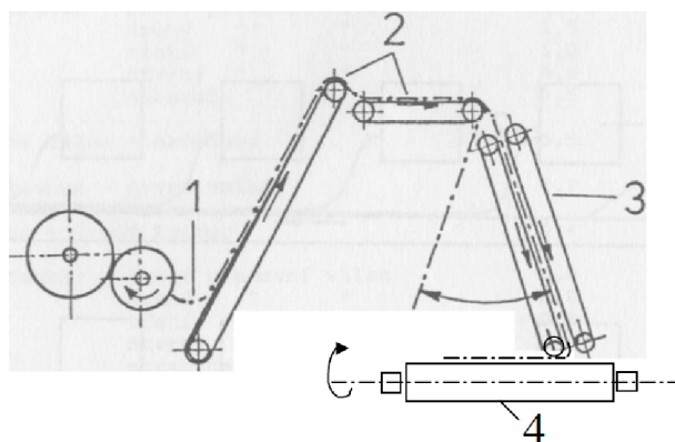
Obr. 5: Schéma vertikálního příčného kladeče pavučiny. 1-pavučina z mykacího stroje, 2- přiváděcí dopravníky, 3-dvojice výkyvných kladečích pásů, 4-odváděcí dopravník [16]
