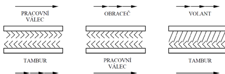
Obr. 4: Znárodnění postavení pracovních povlaků na válcích mykacího stroje [16]
