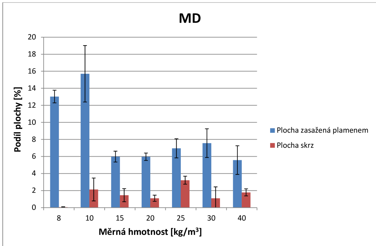
Graf 1 - Zastoupení podílu ploch pro směr výstupu materiálu ze stroje
