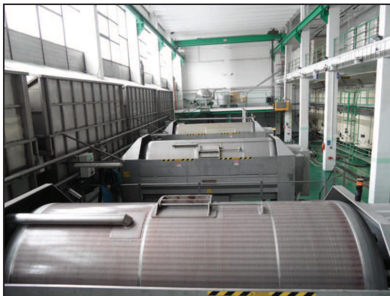
Obr. 6 Pneumatický lis
