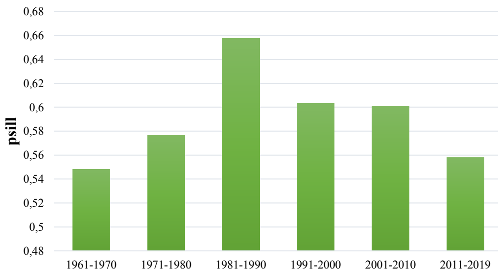
obr. 3.13 Graf odhadované hodnoty psill parametru v jednotlivých desetiletí pro období od 1.1.1961 do 31.12.2019
