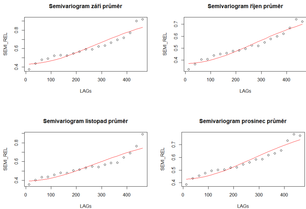
obr. 3.1 Semivariogramy jednotlivých měsíců pro období od 1.11961 do 31.12.2019
