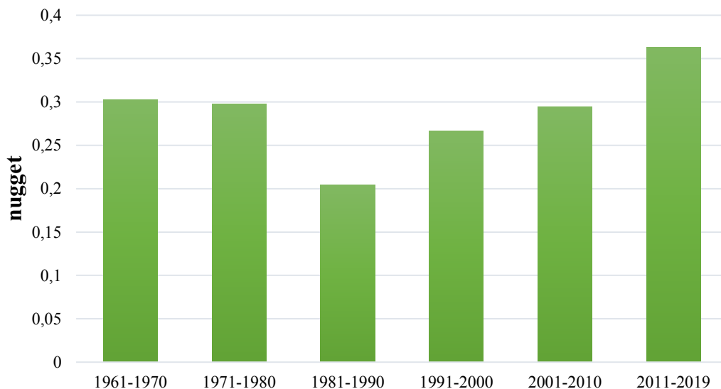
obr. 3.12 Graf odhadované hodnoty nugget parametru v jednotlivých desetiletí pro období od 1.1.1961 do 31.12.2019
