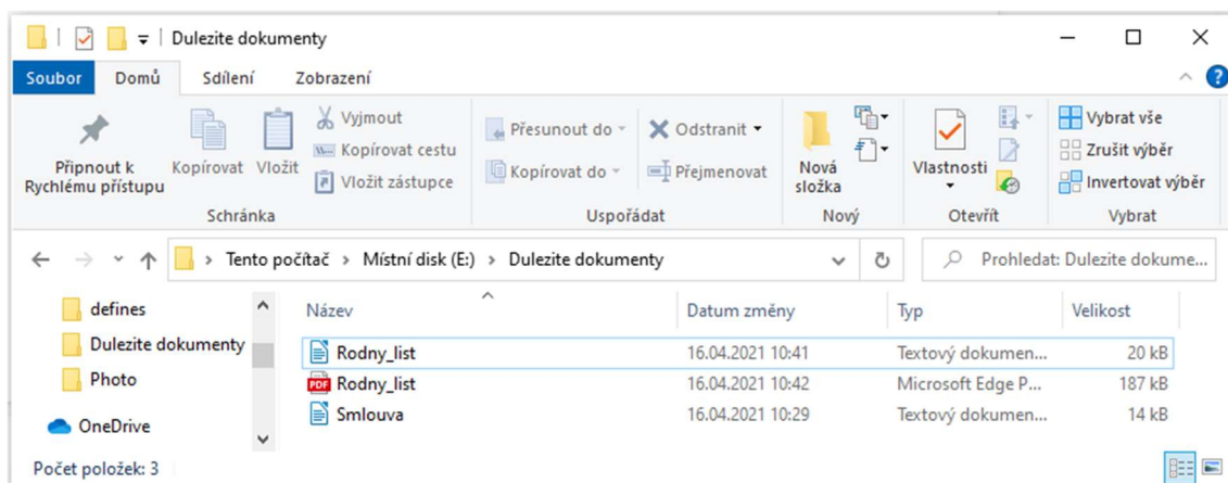
Obrázek 23: Testovací soubory
