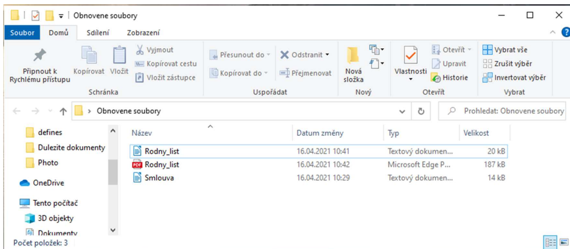
Obrázek 26: Obnovené soubory
