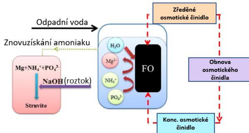
Obr. 4.16 – Schéma OMBR pro recyklaci amoniaku. FO - dopředná osmóza. Převzato a přeloženo z [70].
