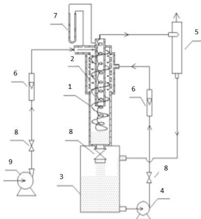
Obr. 4.9 – Experimentální schéma aerocyklónového reaktoru s rozprašováním. 1 – aerocyklona s rozprašovanou vodou; 2 – porézní část reaktoru; 3 – nádrž s vodou; 4 – oběhové čerpadlo; 5 – oddělení plynu od kapaliny; 6 – plovákový průtokoměr; 7 – manometr; 8 – ventil; 9 – vývěva [61].
