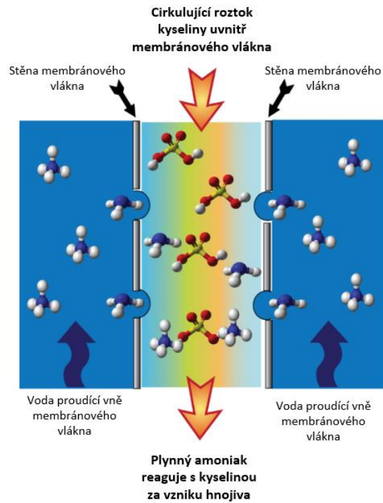
Obr. 4.18 – Schéma vzniku síranu amonného přes membránové vlákno. Převzato a přeloženo z [79].
