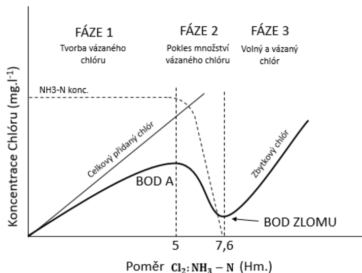
Obr. 4.20 – Diagram znázorňující proces chlorování do bodu zlomu jako závislost koncentrace chlóru a hmotnostního poměru chlóru s amoniakem, převzato a přepracováno [88].
