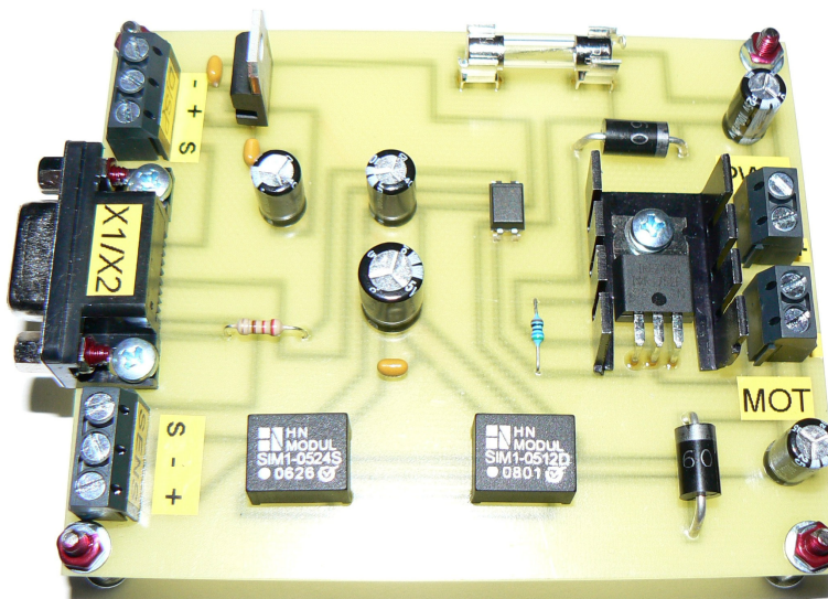
Obr.4.5: Deska plošných spojů komunikační jednotky
