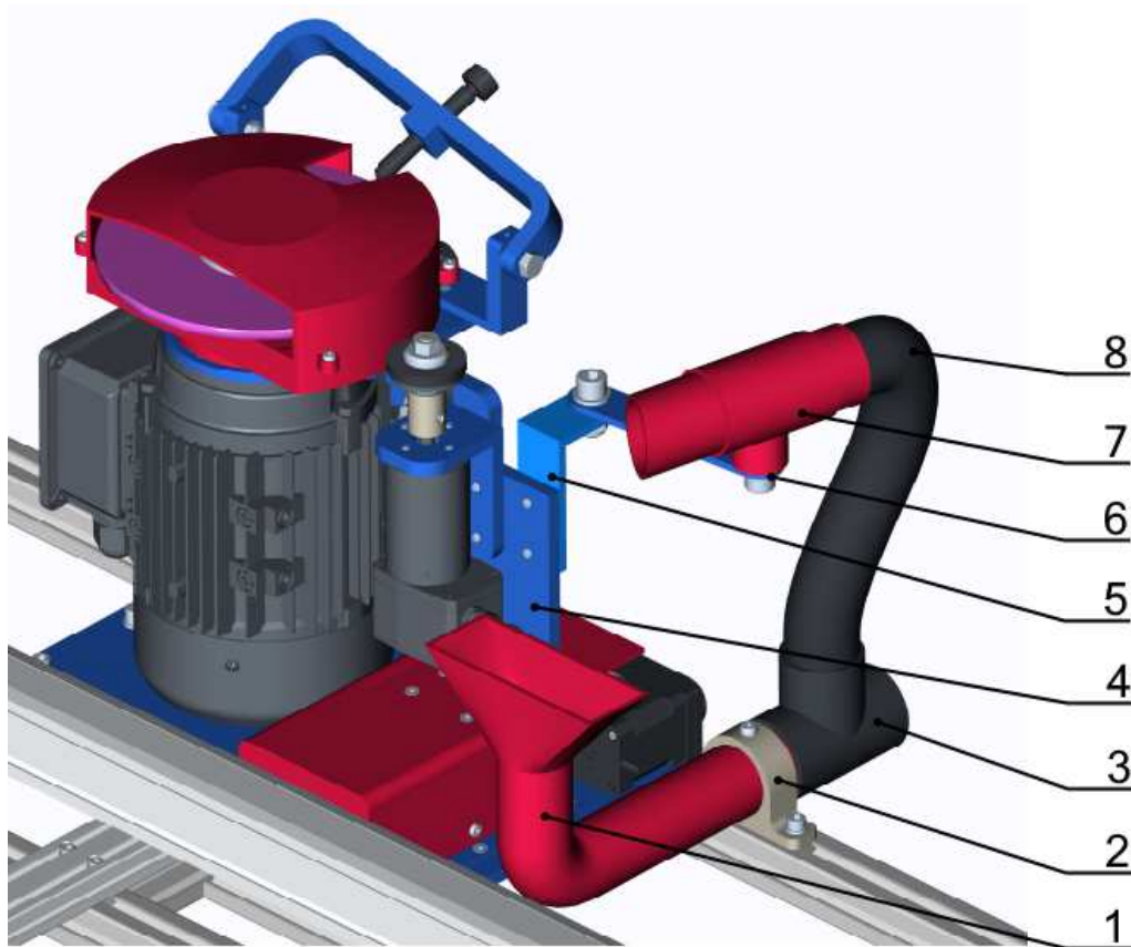
Obr. 2.23 – Odsávání zařízení
