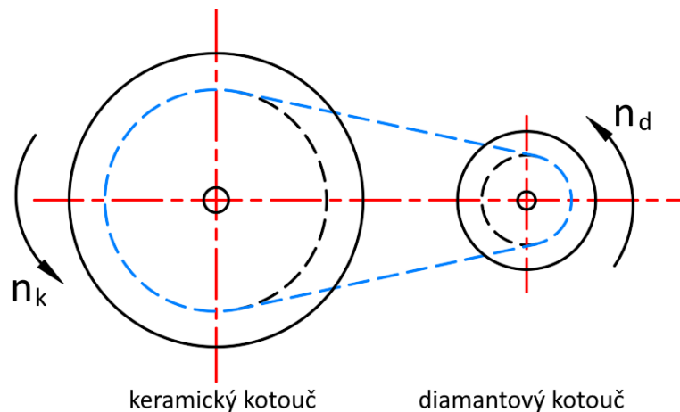
Obr. 2.3 – Návrh varianty 1
