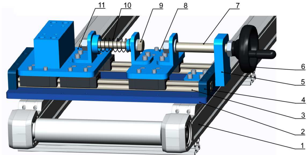
Obr. 2.11 – Příčný pojezd
