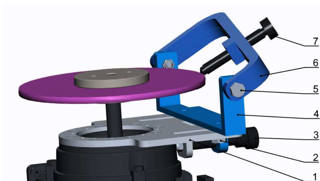
Obr. 2.17 – Orovnávací mechanismus
