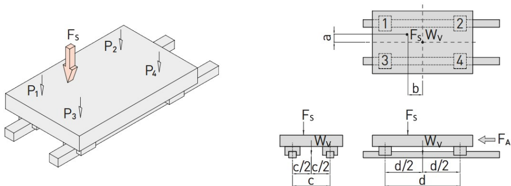
Obr. 2.12 – Zatížení vozíku (statické) [46]
