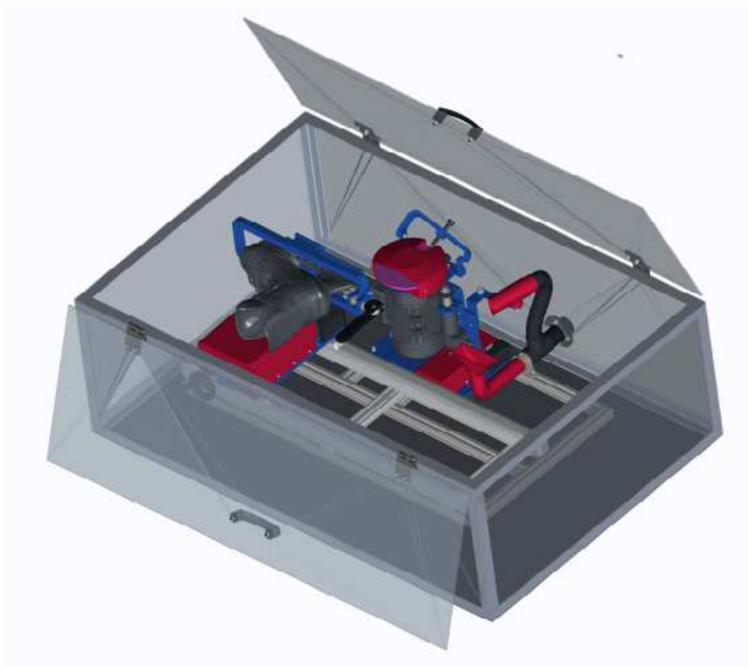
Obr. 2.26 – Uložení zařízení do skříně
