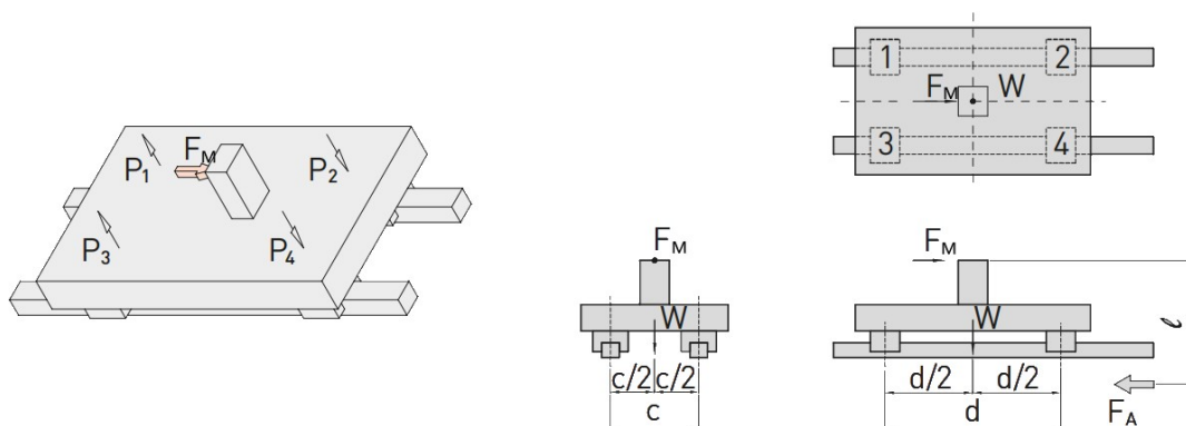
Obr. 2.13 – Zatížení vozíku (pohybové) [46]
