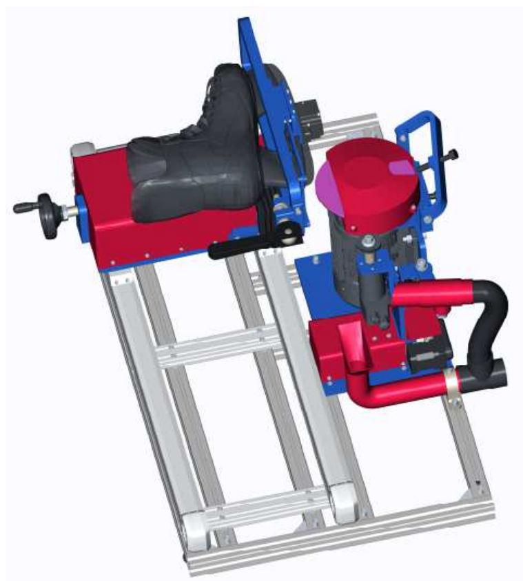
Obr. 2.25 – Model sestavy brousícího zařízení (2)
