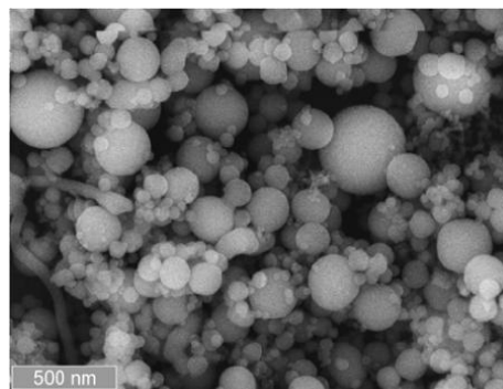
Obrázek 7: SEM snímek mikrosiliky [16]
