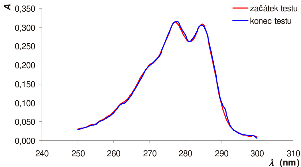
Obr. 27: Porovnání absorpčních spekter 3,5-dichlorofenolu před a po ukončení testu
