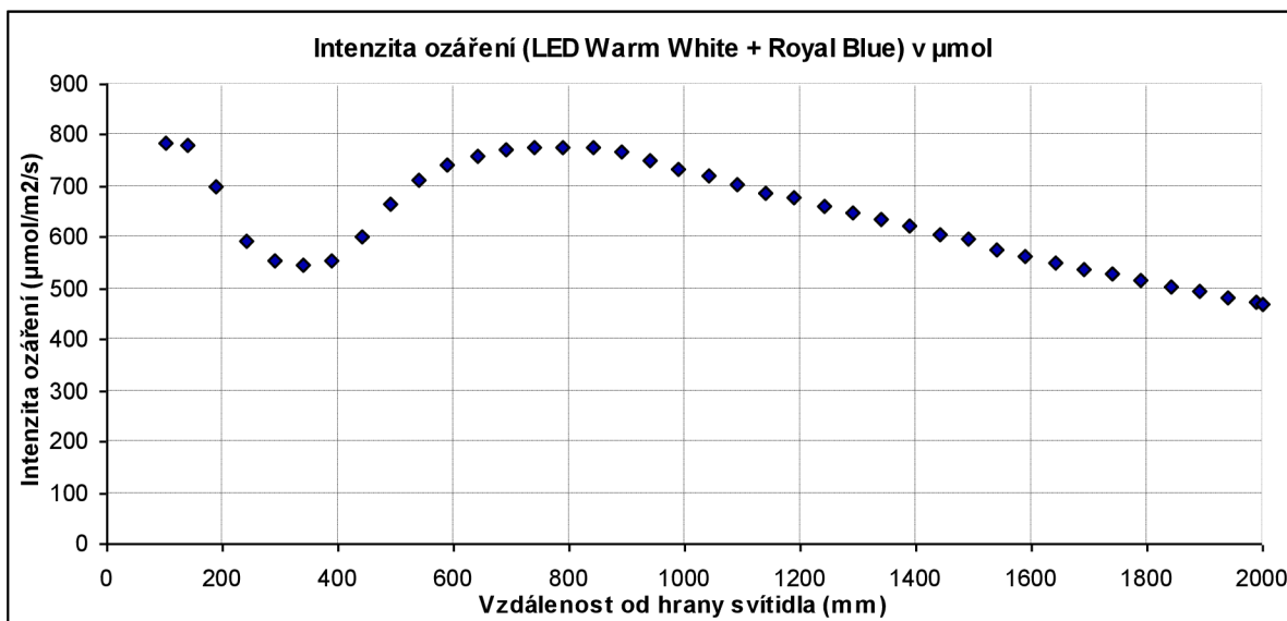
Obr. 5-21 Hodnota intenzity ozáření v \mu\text{mol} – svítilno LED (Warm White + Royal Blue) [18]
