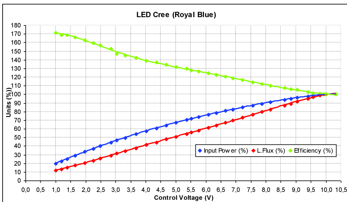
Obr. 5-3 Křížové charakteristiky LED (Royal Blue) [18]
