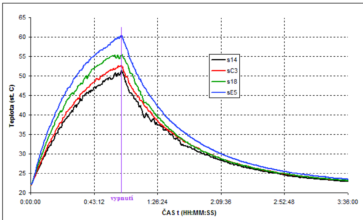
Obr. 5-5 Oteplení LED svítidla bez chlazení [18]
