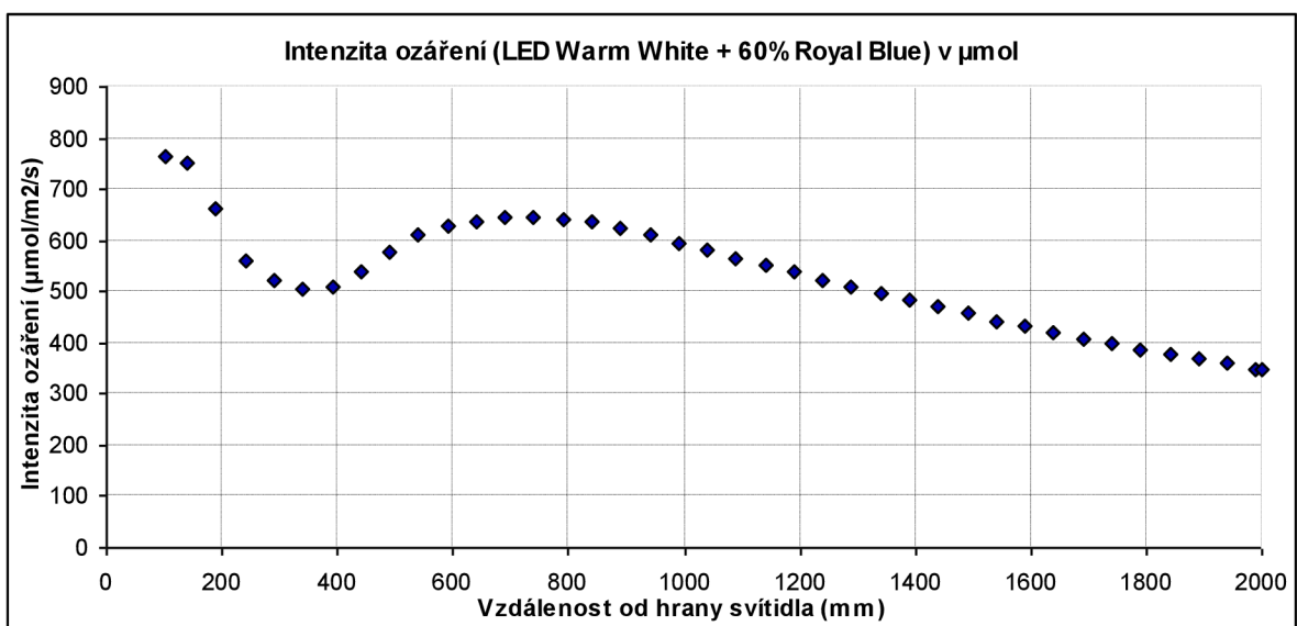
Obr. 5-22 Hodnota intenzity ozáření v \mu\text{mol} – svítilno LED (Warm White + 60 % Royal Blue) [18]
