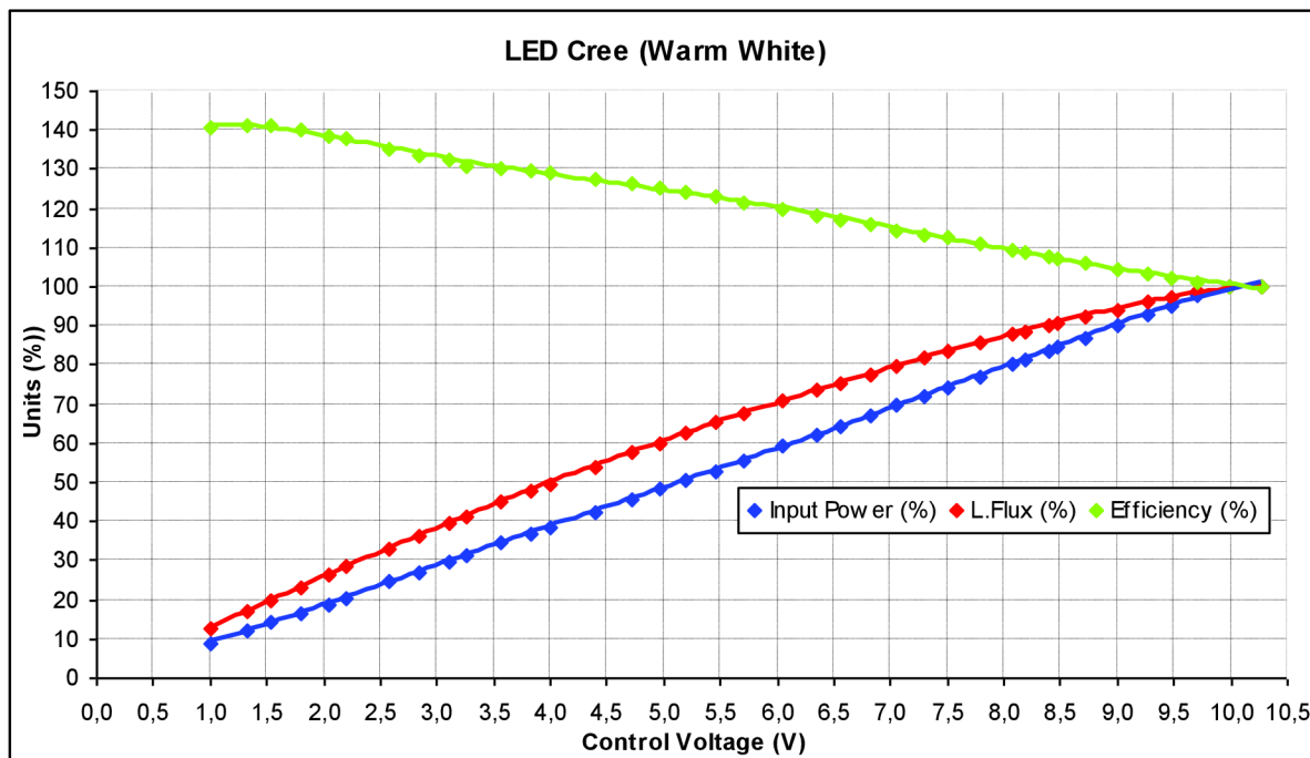
Obr. 5-2 Křížové charakteristiky LED (Warm White) [18]
