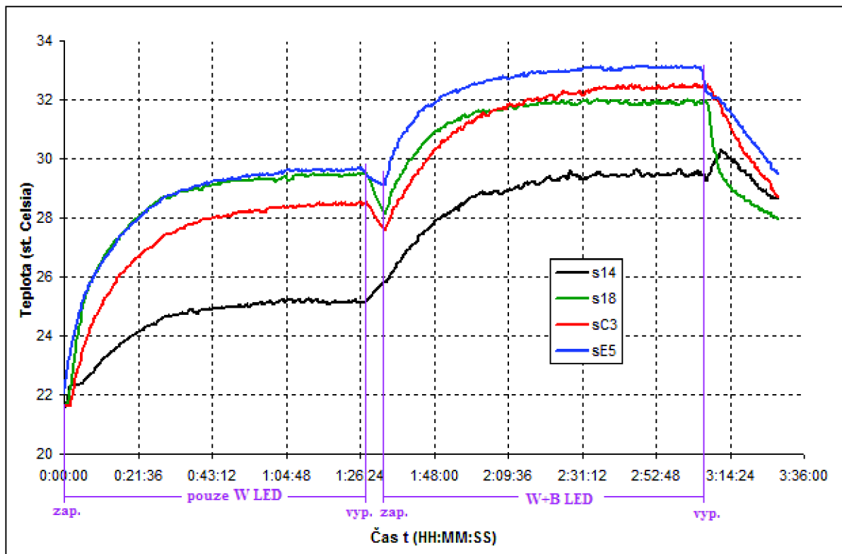
Obr. 5-7 Oteplení LED svítidla s vodním chlazením [18]
