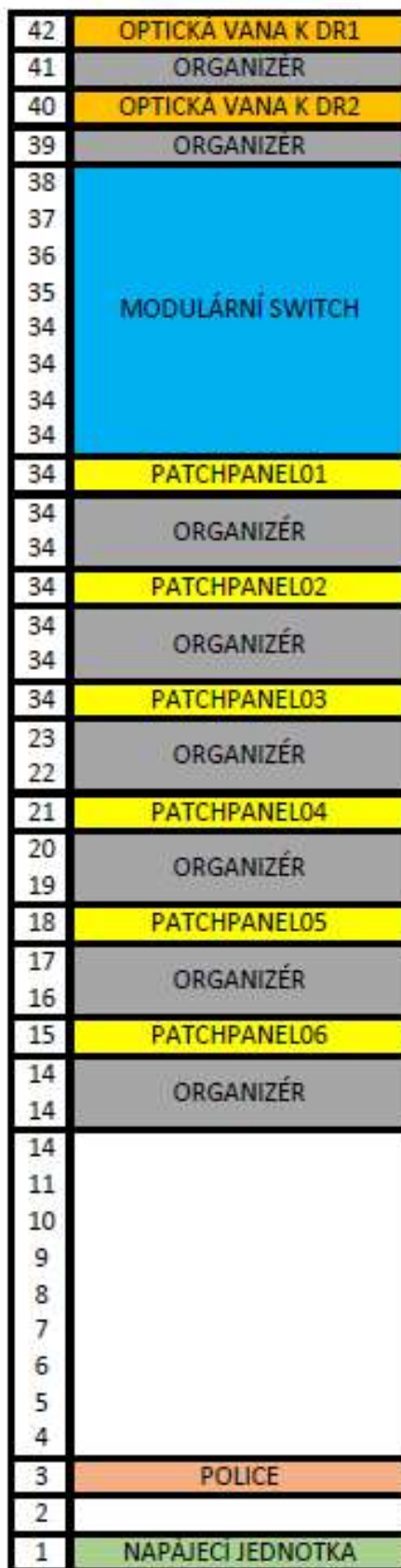
Obrázek 28: Schéma datového rozvaděče (vlastní tvorba)
