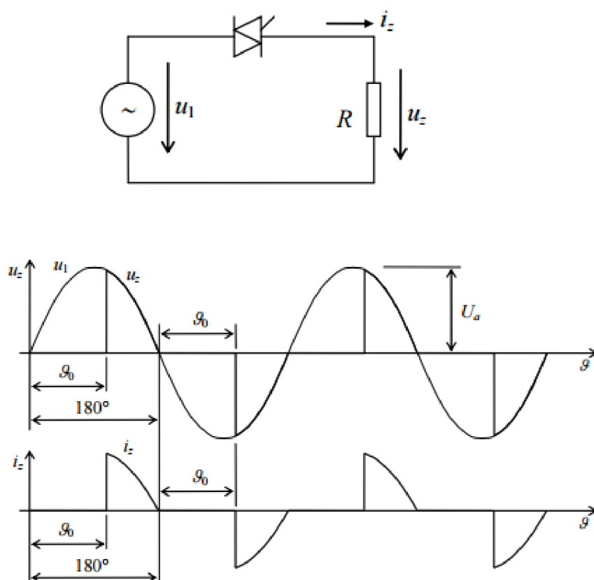
Obr. 4-2: Striedavý menič napätia s odporovou záťažou a priebehy napätia a prúdov [35]
