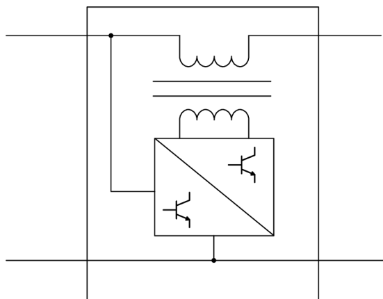
Obr. 4-4: Principiálna schéma sériového transformátora s meničovým buđením [37]
