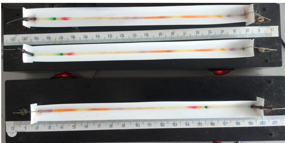
Obrázek 6: Systém mikropreparativní izoelektrické fokusace při separaci
