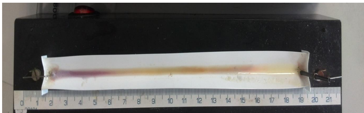
Obrázek 15: Koryto s nadávkovaným roztokem cytochromu c o koncentraci 1 mg/ml a pI markery po 3 hod fokusace
