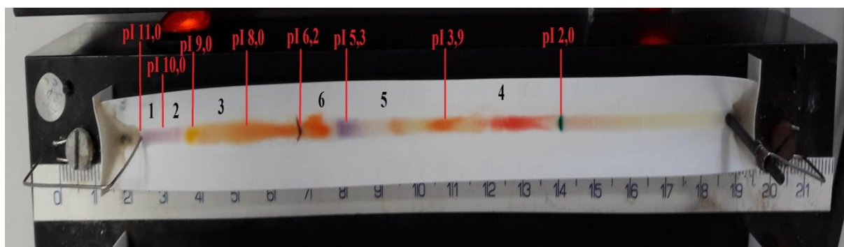
Obrázek 29: Koryto s nadávkovanou směsí roztoku cytochromu c o koncentraci 0,5 mg/ml a roztoku albuminu o koncentraci 0,5 mg/ml a pI markery po 24 hod fokusace
