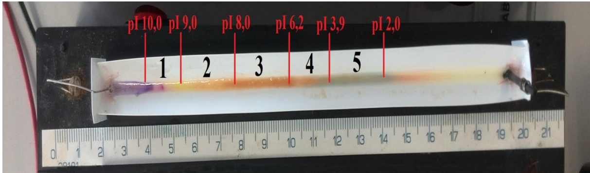
Obrázek 16: Koryto s nadávkovaným roztokem cytochromu c o koncentraci 1 mg/ml a pI markery po 6 hod fokusace
