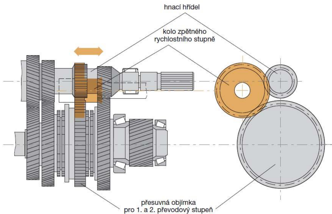
Obr. 3.25 Řazení zpětného chodu převodovky 02K [14]
