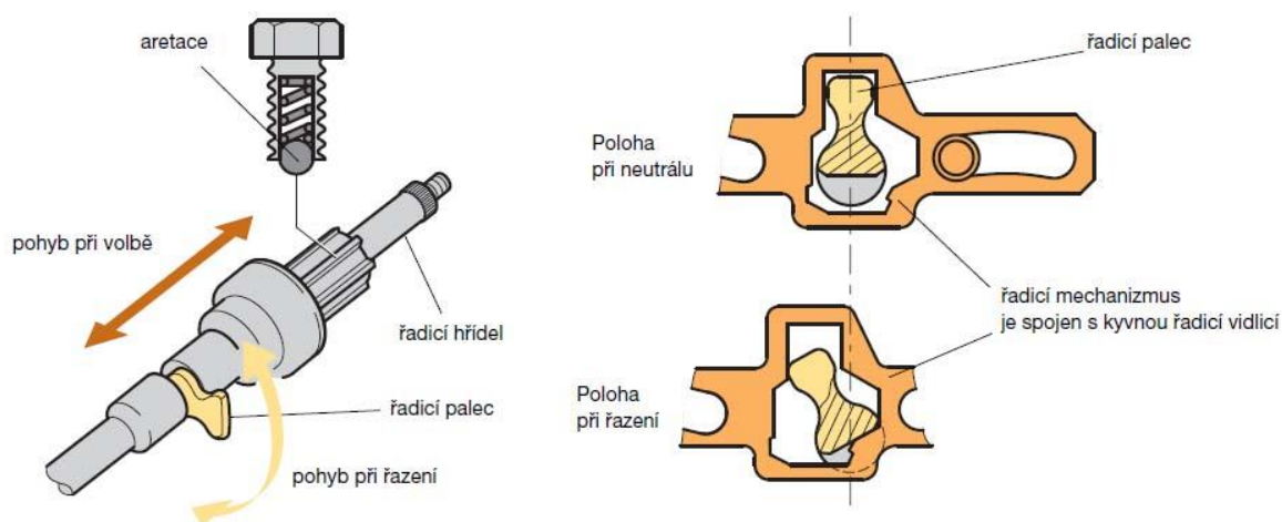
Obr. 3.16 Proces řazení převodovky 02J [14]
