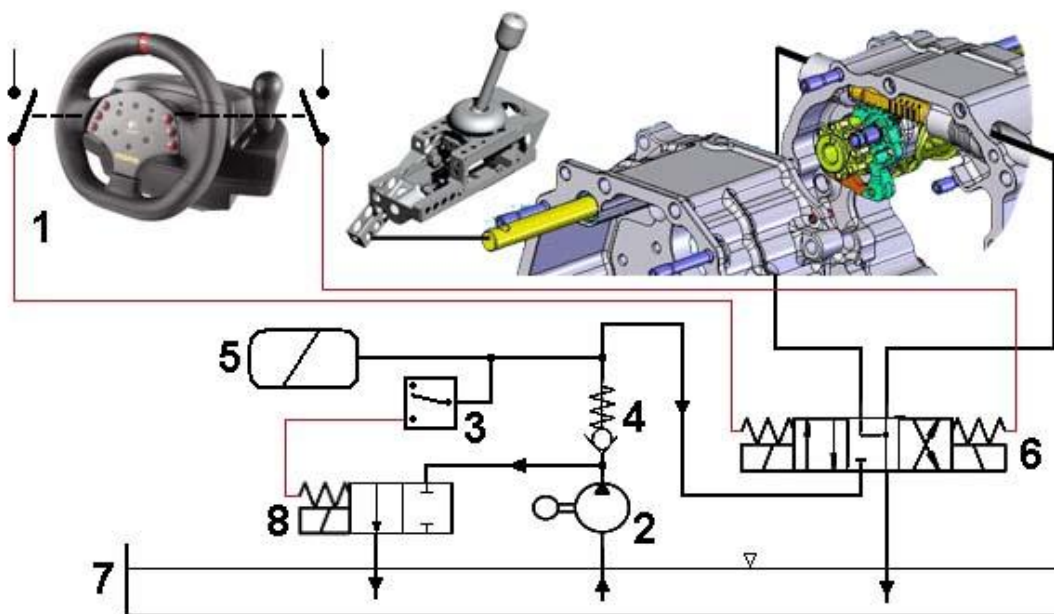
Obr. 3.24 Schéma hydraulického ovládání sekvenční převodovky Kaps Transmission [15]
