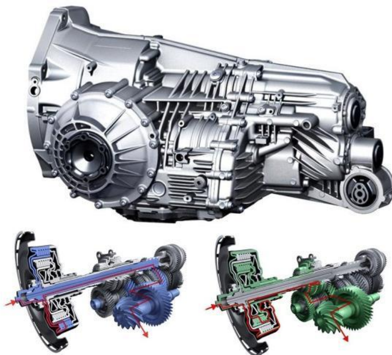
Obr. 4.6 PDK převodovka od Porsche [23]
