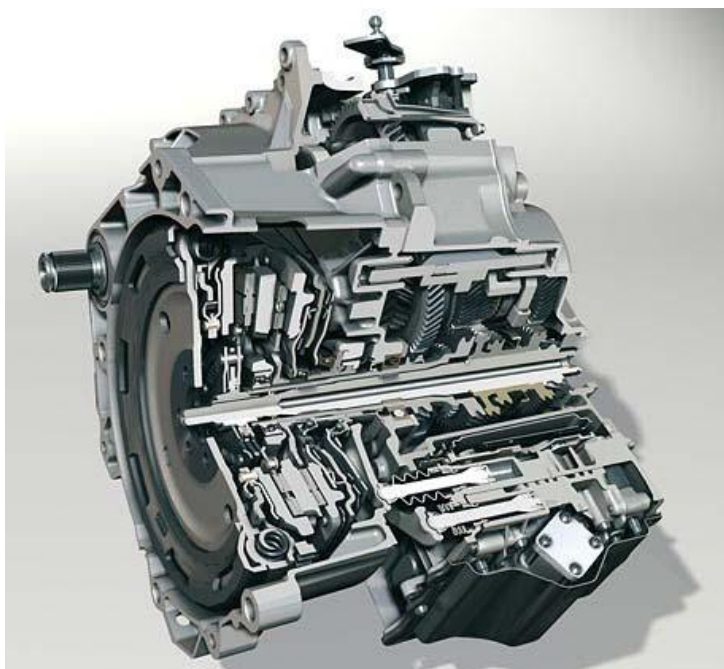
Obr. 4.5 Přebodovka DSG-7 pro příčnou zástavbu [22]
