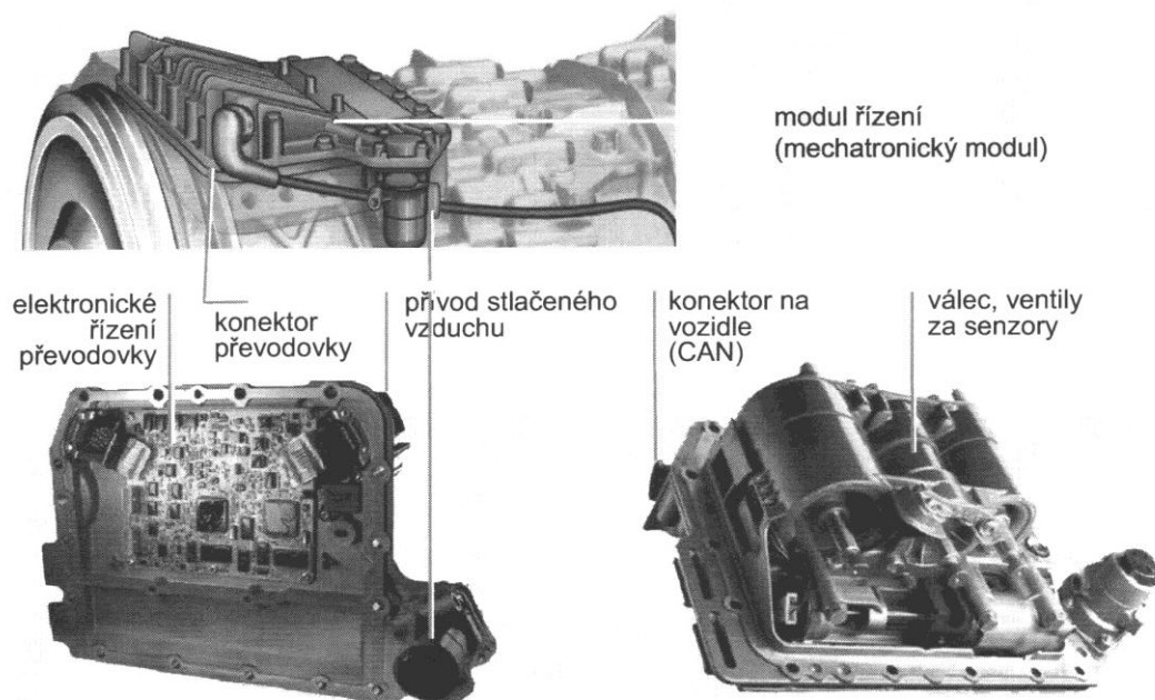
Obr. 3.23 Mechatronický modul elektropneumatického ovládní převodovky ZF-AS Tronic [16]
