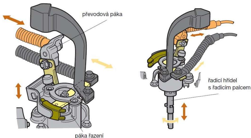
Obr. 3.22 Převod řadičího a voličiho pohybu na víku převodovky [14]
