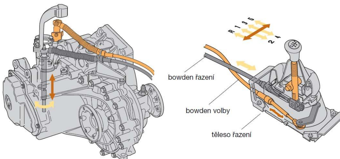
Obr. 3.20 Lanový převod ovládacích pohybů převodovky 02J [14]
