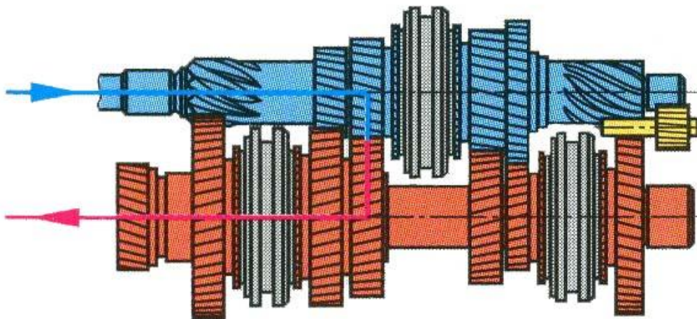
Obr. 2.1 Schéma dvouhřídelové převodovky [9]
