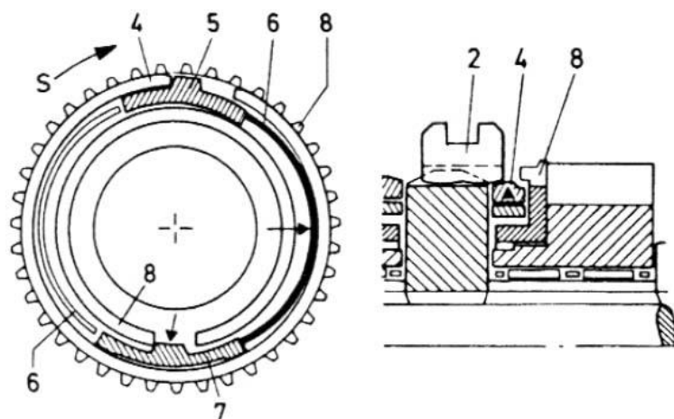
Obr. 3.9 Činnost blokovací synchronizace: 2- řadicí objímka; 4- synchronizační kroužek; 5- kámen; 6- blokovací pásek; 7- doraz; 8- těleso spojky; [12]
