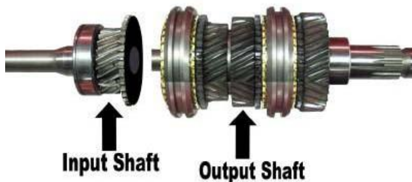
Obr. 2.3 Uložení výstupního a vstupního hřídele [10]
