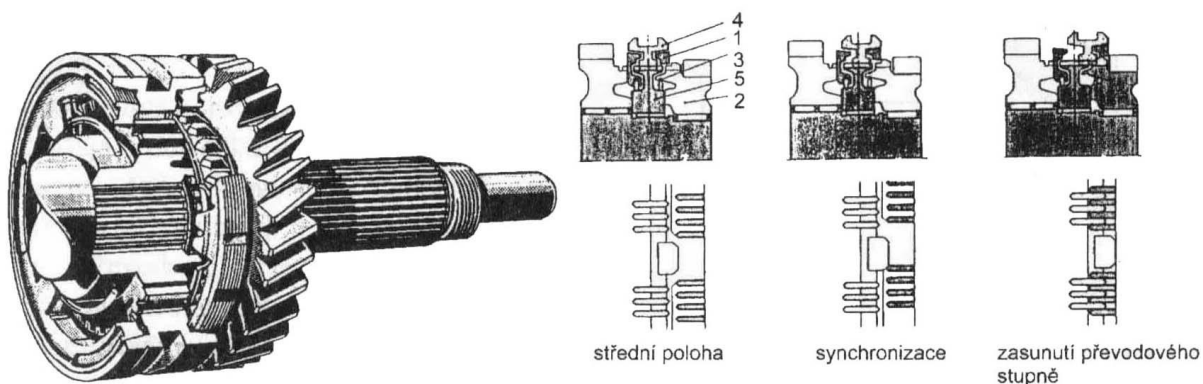
Obr. 3.6 Vnější synchronizace: 1 – clonící kroužek; 2 – ozubené kolo; 3 – prstencová pružina; 4 – řadicí objímka; 5 – těleso řadicí objímky [3]
