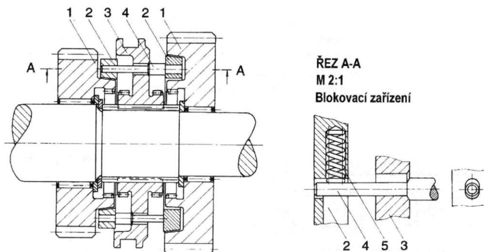
Obr. 3.10 Synchronizace s blokujícím čepem: 1- ozubené kolo; 2- synchronizační kroužek; 3- řadicí objímka; 4- blokovací čep; 5- tlačná pružina [3]
