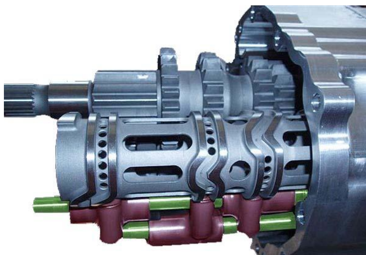
Obr. 3.18 Řadicí válec převodovky Kaps Transmission [15]
