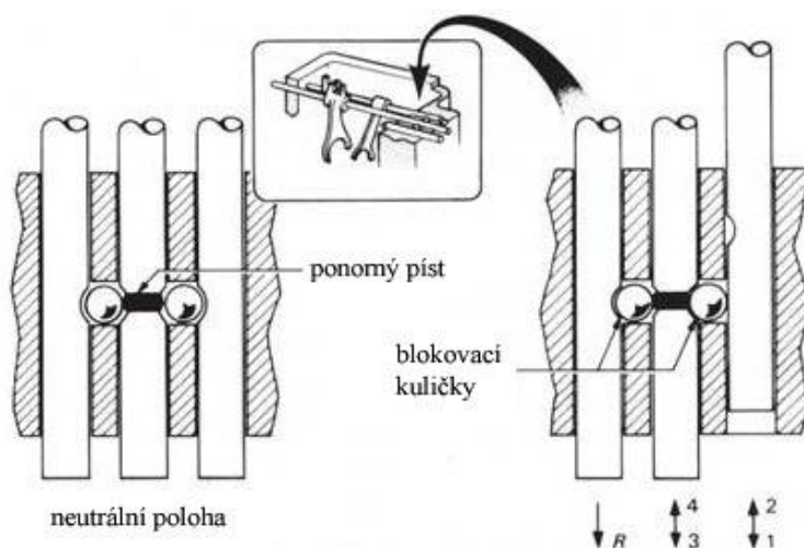
Obr. 3.13 Zajišťovací zařízení [13] (obrázek opatřen českými popisky)
