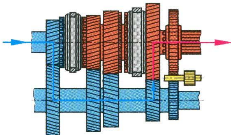
Obr. 2.2 Schéma tříhřídelové převodovky [9]
