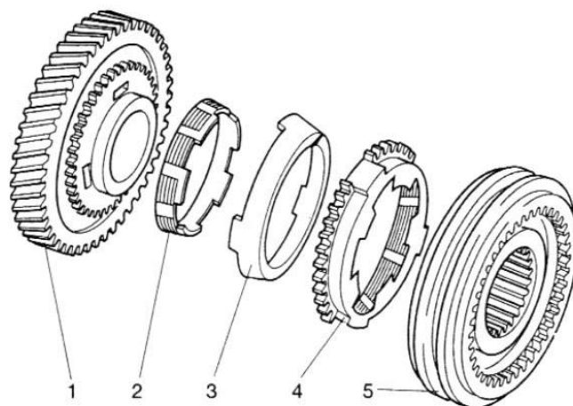
Obr. 3.5 Dvojitá synchronizace: 1- ozubené kolo převodu; 2- vnitřní synchronizační kroužek; 3- vnější prstenec; 4- vnější synchronizační kroužek; 5- řadicí objímka s tělesem [12]
