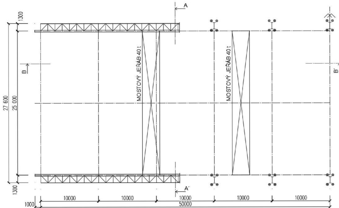
Obr. 1.3. – Dispozice konstrukce – půdorys
