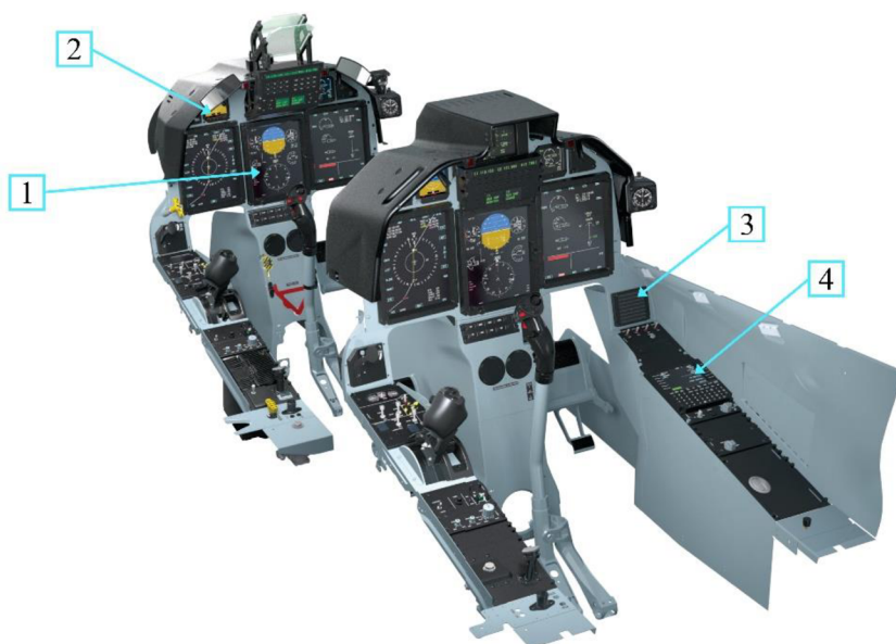
Obrázok 3.4 Kabína PC-21 [10]
