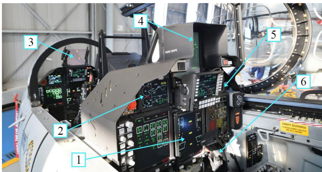
Obrázok 3.2 Kabína M-345 [23]
