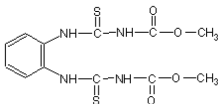
Obr. 5: Strukturní vzorec thiofanát-methylu.
