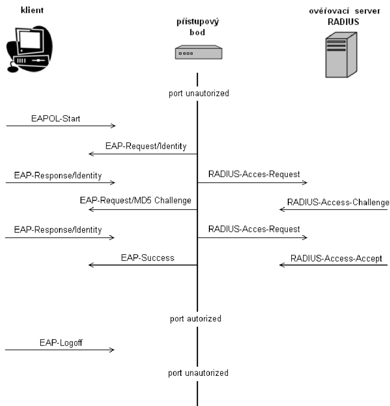
Obrázek 4.3: 802.1x autentizace
