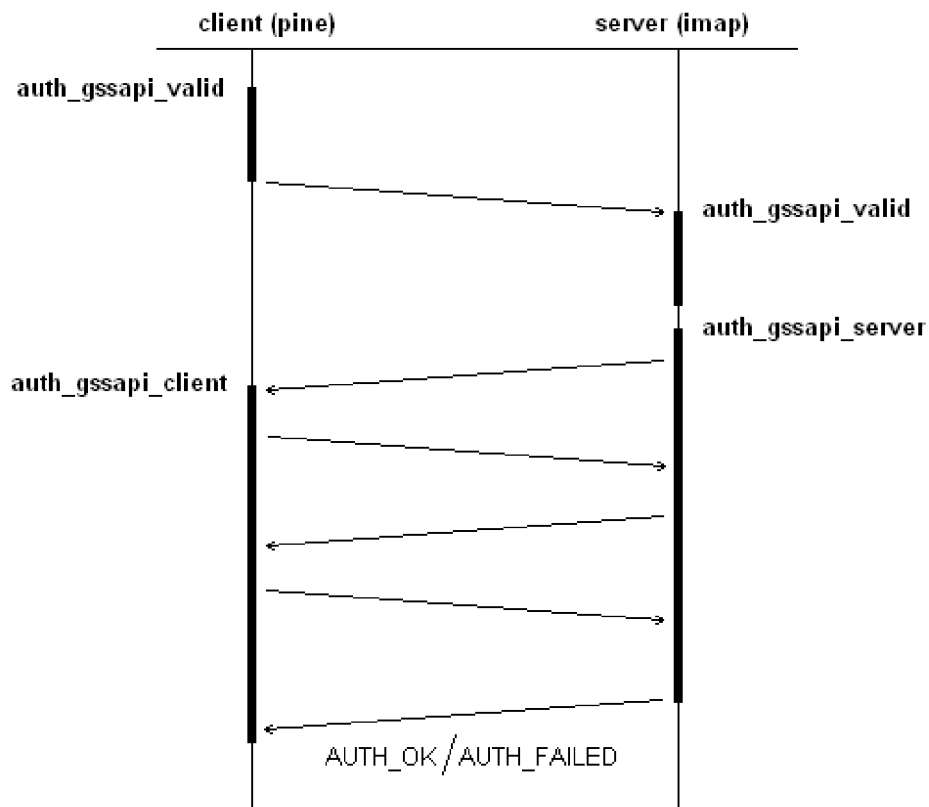
Obrázek 6.2: Atentizace GSSAPI - časový diagram
