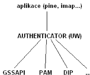
Obrázek 8.1: Nová hierarchie autentizačních vrstev
