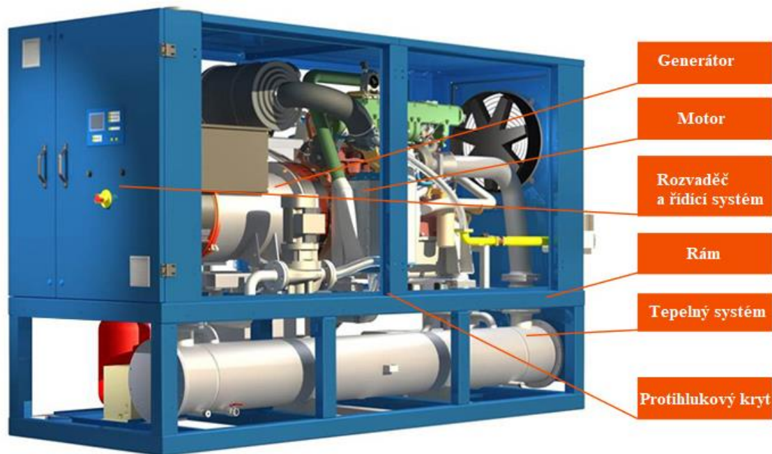
Obr. 2.3 Kogenerační jednotka [17]
