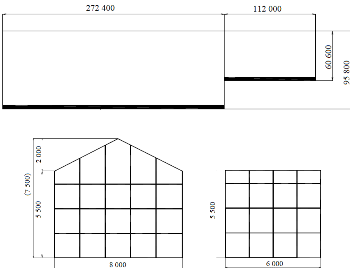
Obr. 3.2. Rozměry skleníku
