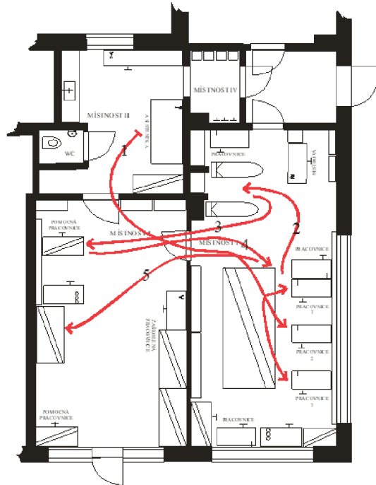
Obrázek 14 Materiálový tok polotovaru B
