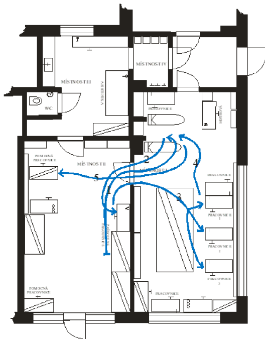
Obrázek 13 Materiálový tok polotovaru A
