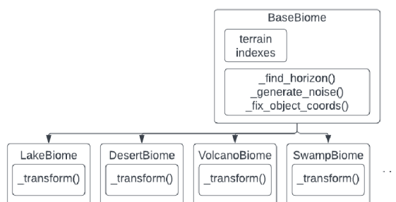
Obrázek 3.6: Objektová reprezentácia štruktúry biómových modulov.
