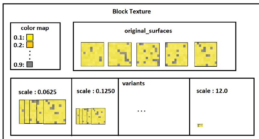
Obrázek 4.12: Vnútroštruktúra textúry pre blok. V atribúte original sú uložené textúrové reprezentácie bloku v základnej veľkosti (12×12 pixelov), variants obsahuje transformované textúry do všetkých možných veľkostí v závislosti od zoomu ( scale )
