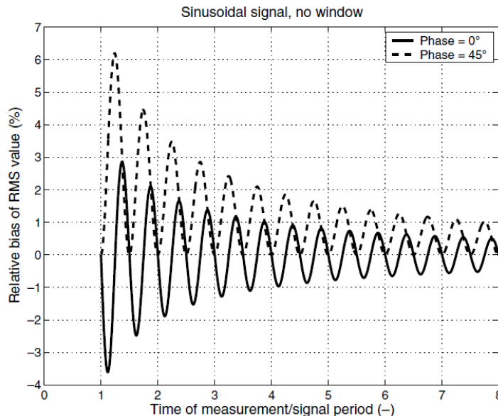
Obrázek 11: Teoretická závislost relativní chyby pro sinusový průběh při použití klasické metody [2]
