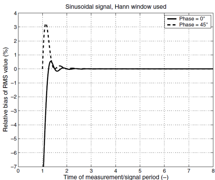
Obrázek 13: Teoretická závislost relativní chyby pro sinusový průběh při použití modifikované metody [2]
