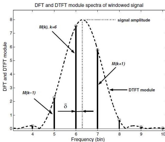
Obrázek 16: Princip interpolace [2]
