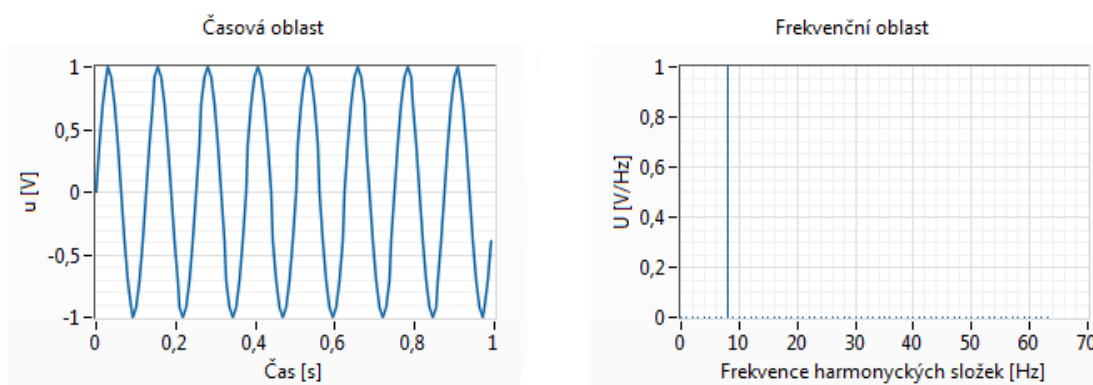
Obrázek 4: Koherentní napět'ový průběh v časové a frekvenční oblasti
