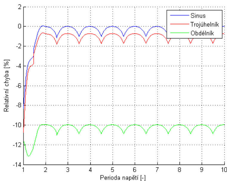
Obrázek 49: Chybová charakteristika pro sinusový, trojúhelníkový, obdélníkový a pilový průběh při stanovení RMS ze spektra s využitím metody oken
