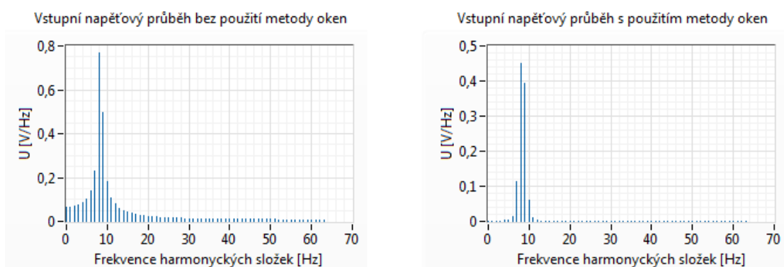
Obrázek 7: Použití metody oken u nekoherentního napěťového průběhu ve frekvenční oblasti
