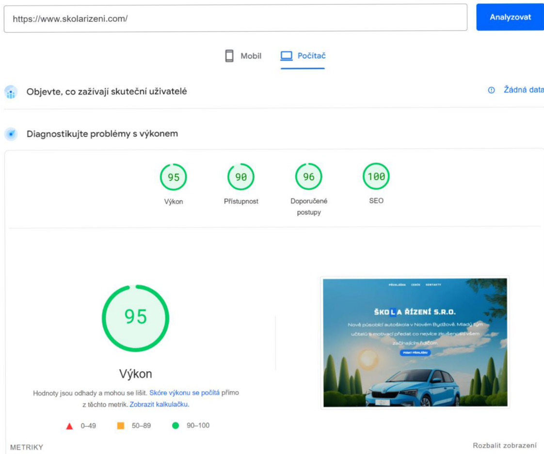
Obrázek 18 PageSpeed Insights, 18. 2. 2024
