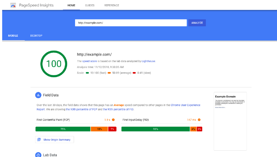
Obrázek 8 PageSpeed Insights
