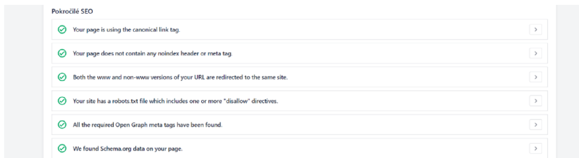
Obrázek 20 PageSpeed Insights, 18. 2. 2024
