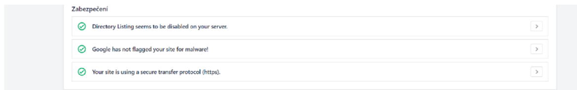
Obrázek 21 PageSpeed Insights, 18. 2. 2024
