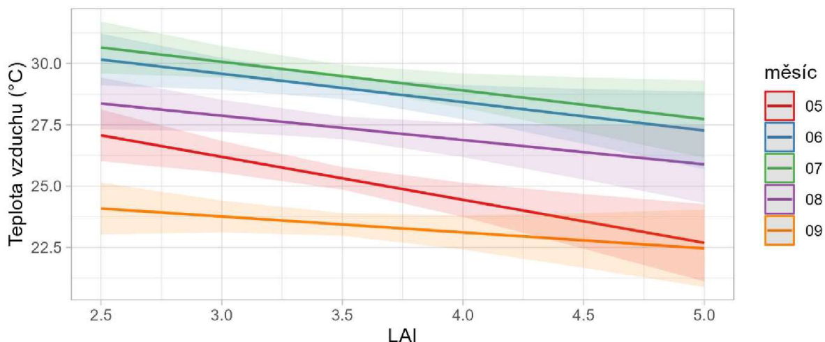
Obrázek 30: Závislost průměrné hodnoty denního maxima teploty vzduchu ve vegetačním období (květen-září) na LAI.
