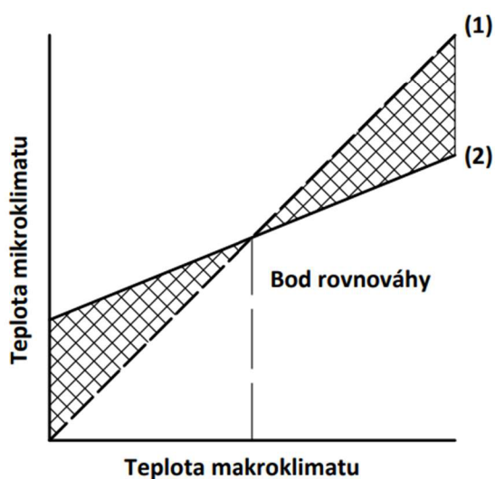
Obrázek 1: Závislost teploty makroklimatu na potlačení teplotních výkyvů lesním ekosystémem. (1) Křivka závislosti bez vlivu lesa ( T. \text{makro} = T. \text{mikro} ). (2) Křivka závislosti při ovlivnění lesním ekosystémem. Bod rovnováhy je stav, při kterém je teplota v porostu rovna teplotě mimo něj. Šrafovaná plocha znázorňuje rozdíl teploty makroklimatu a mikroklimatu (De Frenne et. al., 2021).
