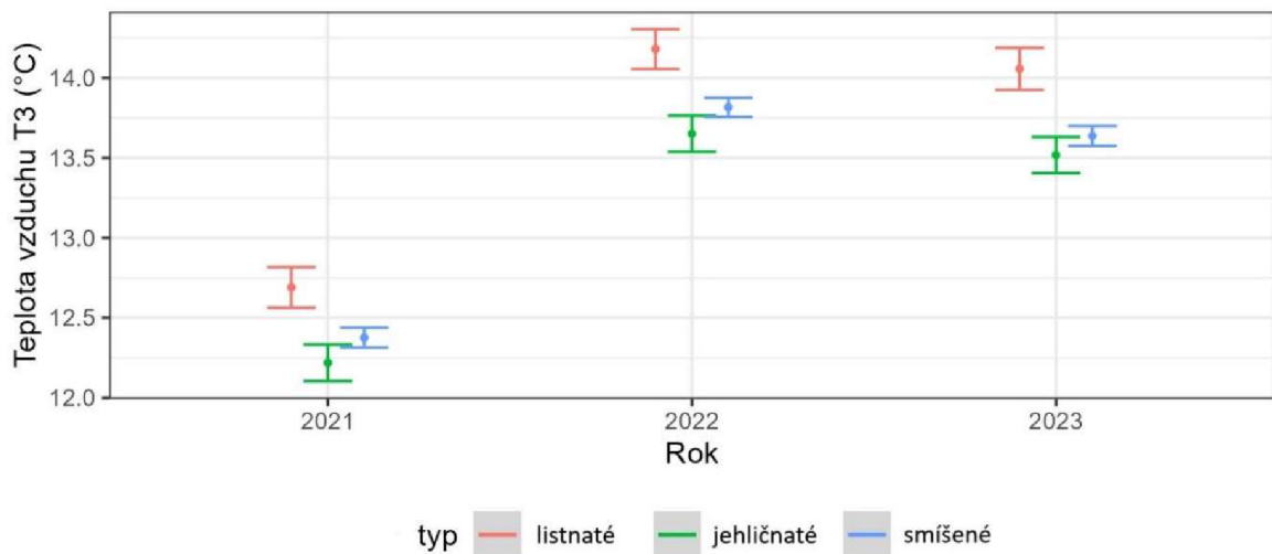
Obrázek 2712: Průměrná teplota vzduchu ve vegetačním období jehličnatých, listnatých a smíšených porostů s 95 % intervalem spolehlivosti.
