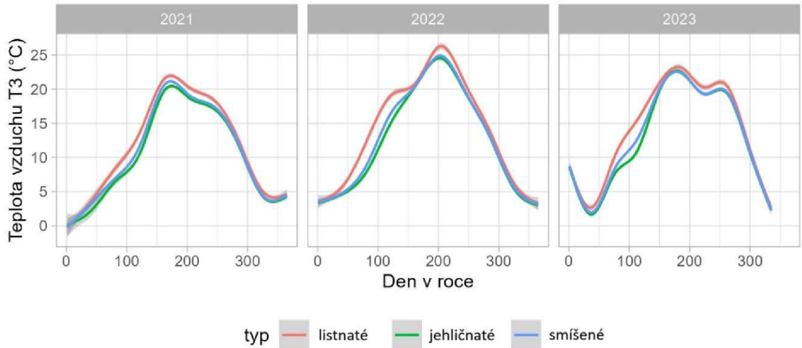
Obrázek 26: Průběh maximální denní teploty vzduchu jehličnatých, listnatých a smíšených porostů v letech 2021–2023.
