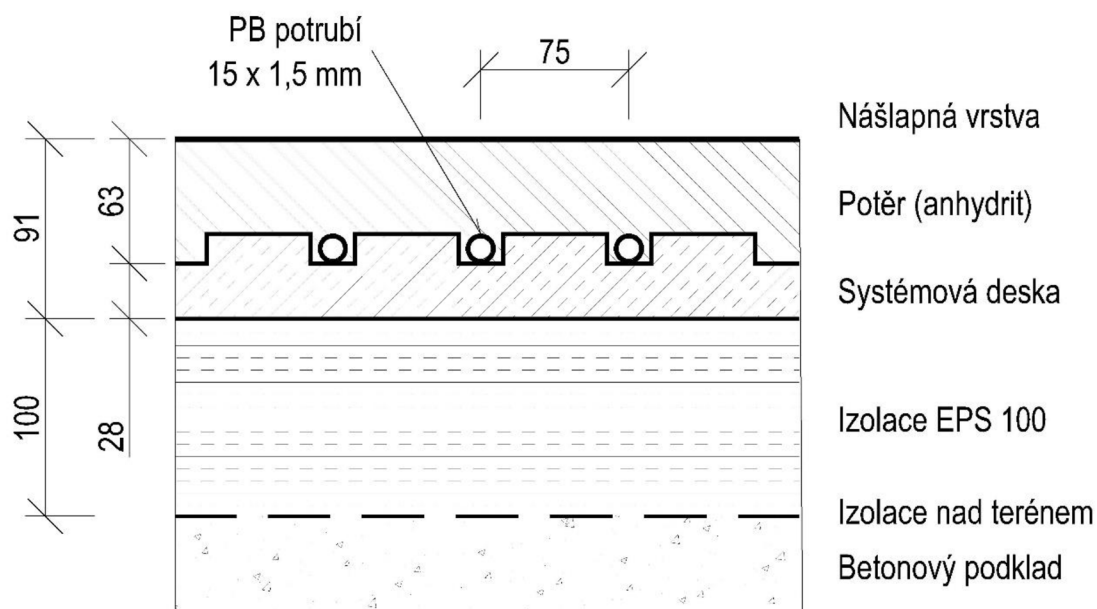
Obr. 2.3 podlahová konstrukce s vytápěním
