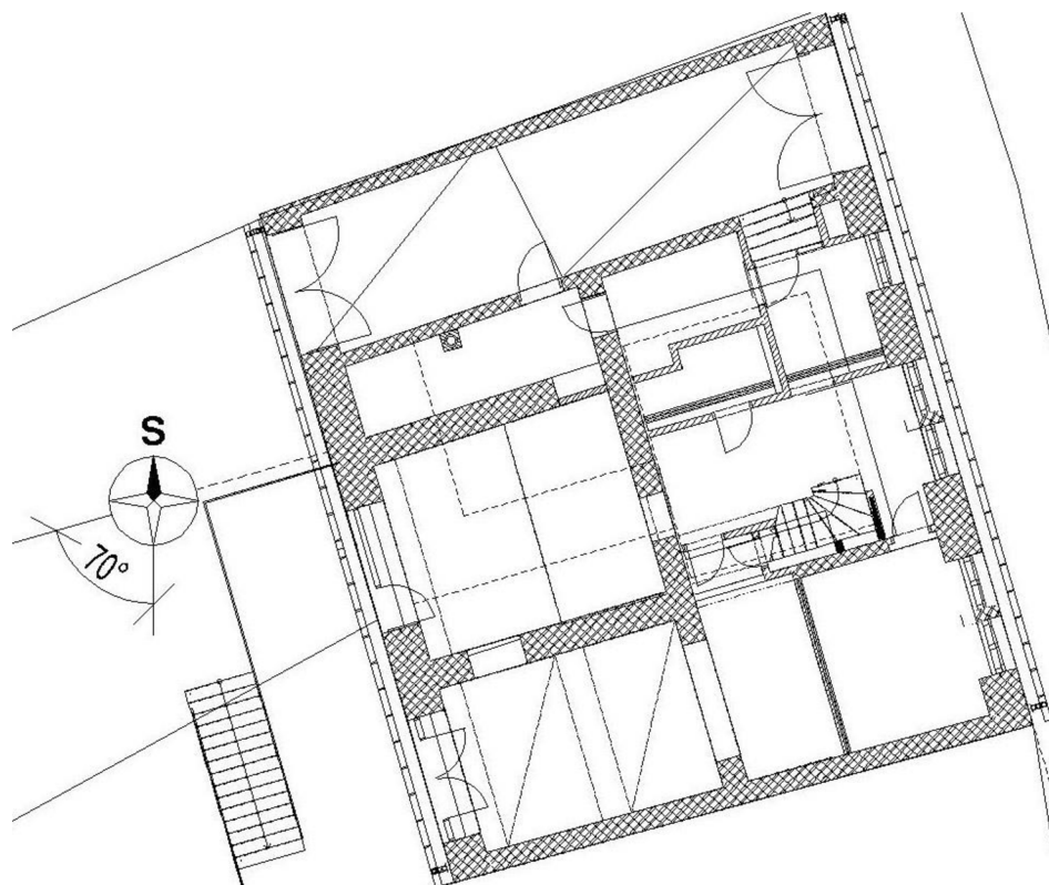
Obr. 2.15 situační náčrtek řešeného objektu
