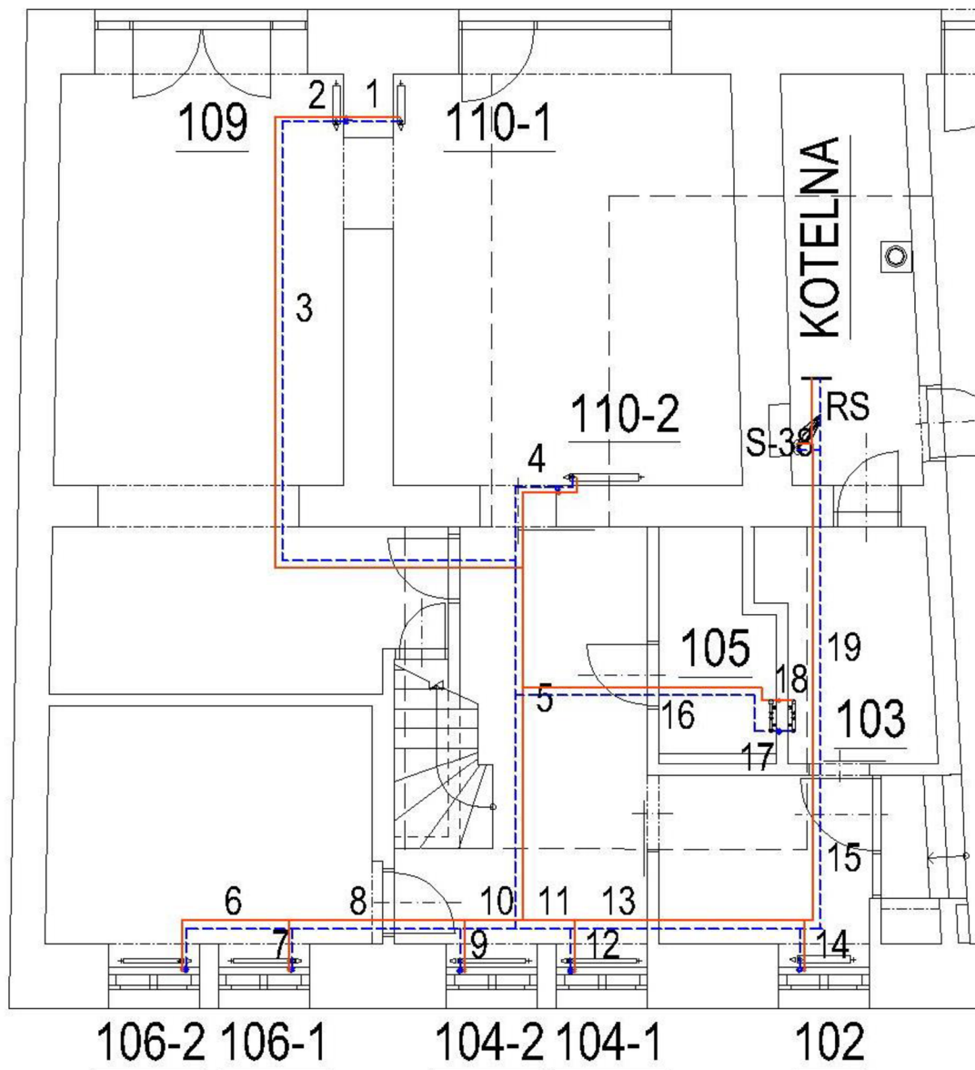
Obr. 2.11 přehledové schéma vytápění otopnými tělesy v 1.NP
