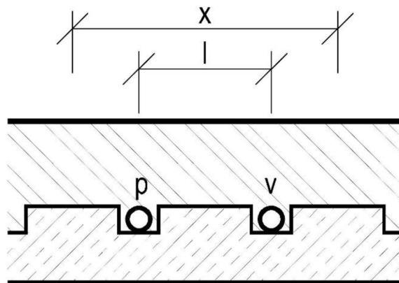
Obr. 2.5 šířka plochy přípojky
