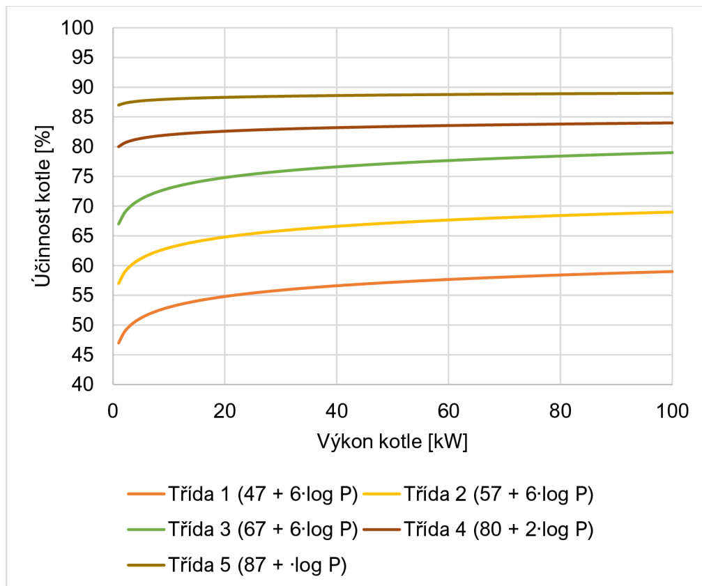
Obr. 1.3 požadavky na minimální účinnosti jednotlivých tříd kotlů v závislosti na jmenovitém výkonu dle [8] [7]
