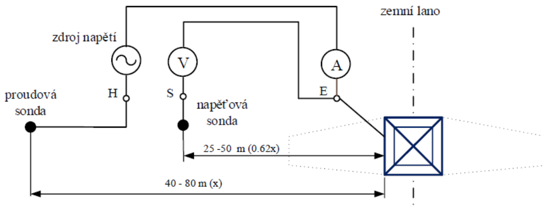
Obrázek 3.11 3 - pólová metoda [5]
