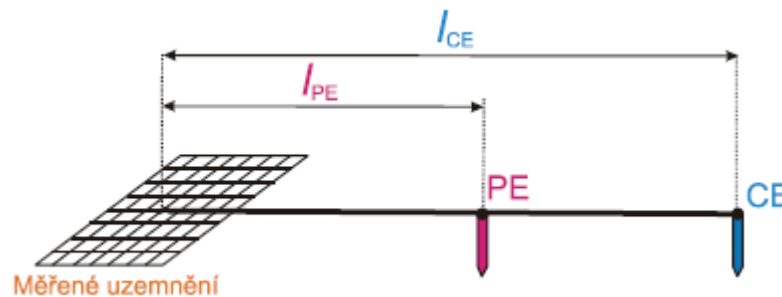
Obrázek 3.4 Rozmístění PE a CE elektrod, vzdálenost l_{PE} = 0,625 \cdot l_{CE} [8].
