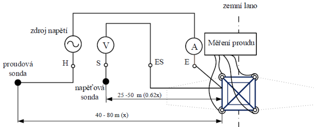
Obrázek 3.10 4 - pólová metoda 62 % [5]
