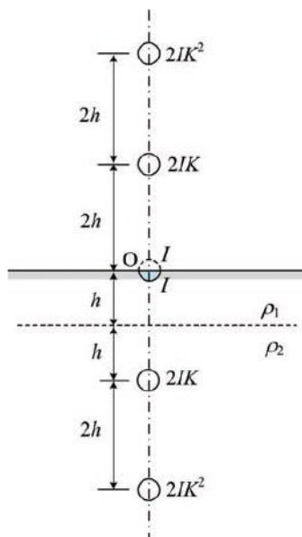
Obrázek 1.5 Hemisférické uzemňovací zařízení a jeho obrazy ve dvouvrstvé půdě [2].
