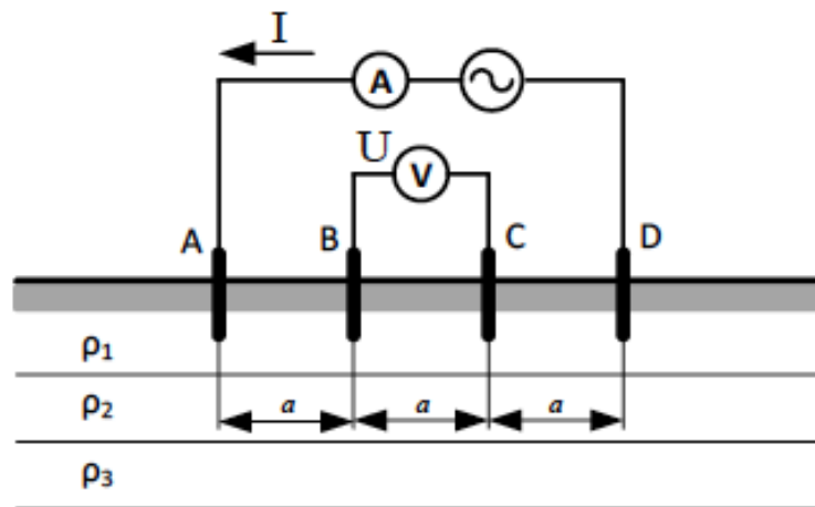
Obrázek 2.1 Schéma konfigurace obvodu pro měření rezistivity půdy Wennerovou metodou [5].
