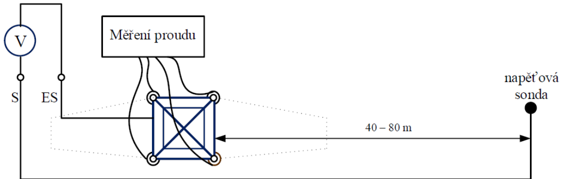
Obrázek 3.12 Pasivní metoda [5]
