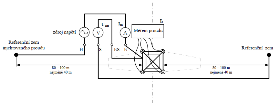
Obrázek 3.9 4 - pólová metoda [5]
