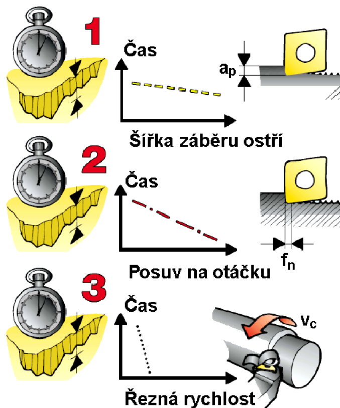
Obr. 4.2 Úspory výrobních nákladů zvýšením řezných podmínek 16
