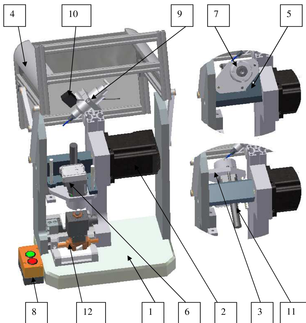
Obr. 16: Náhled na montážní přípravek č.2
