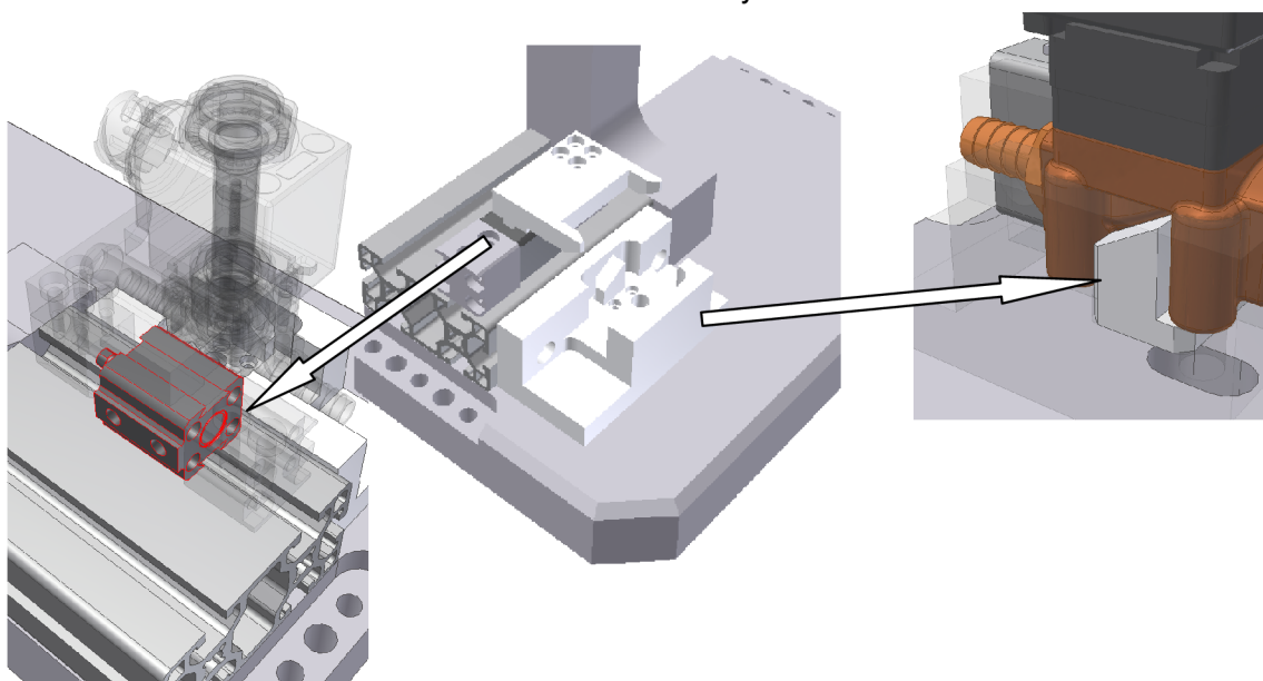
Obr. 25: Orientace konektoru cívky
