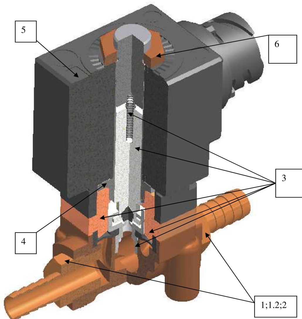
Obr. 9: Řez ventilem
