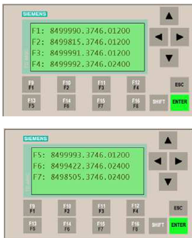
Obr. 22: Volba typu vyráběného ventilu na ovládacím panelu [13]
