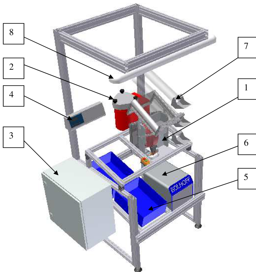
Obr. 17: Náhled celku montážní linky č.2
