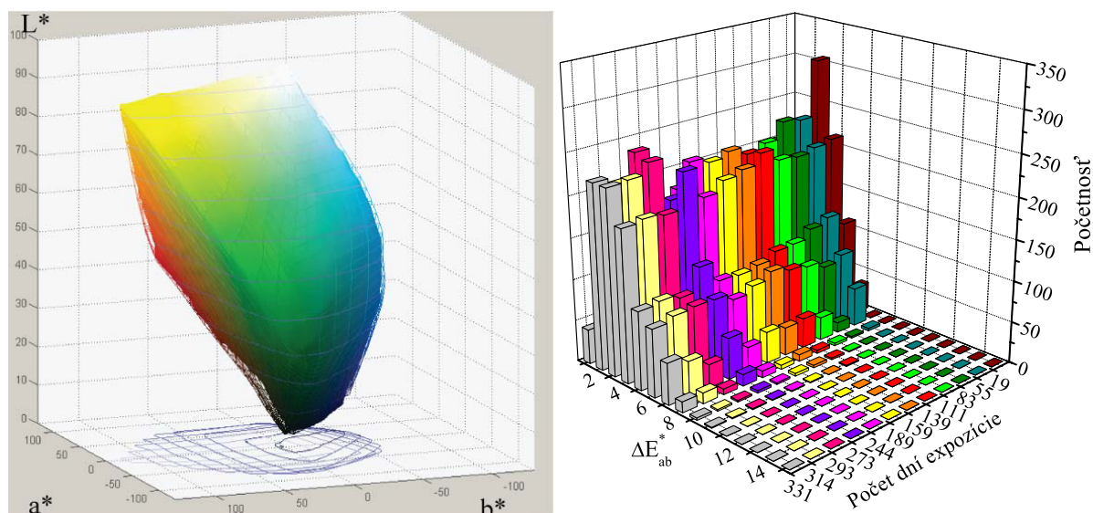
Obr. 91 Vľavo: zmena objemu farbového gamutu testovacej škály na papieri Ilford Classic Gloss, umiestnenej v ráme bez skla. Pred expozíciou (siet') a po expozícii (plný objem). Vpravo: početnosť farbových odchýlok (viď Tabuľka 13).
