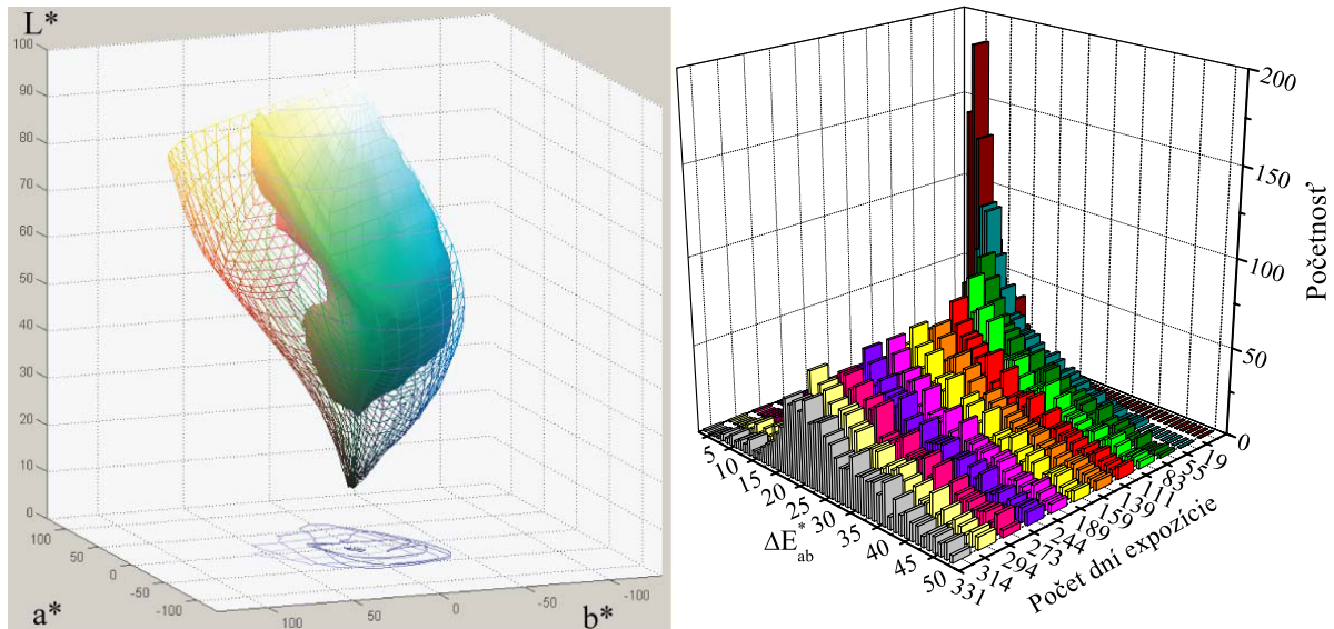
Obr. 79 Vľavo: zmena objemu farebného gamutu testovacej škály na papieri Foma 1224, umiestnenej v ráme bez skla. Pred expozíciou (sieť) a po expozícii (plný objem). Vpravo: početnosť farebných odchýlok (viď Tabuľka 11).
