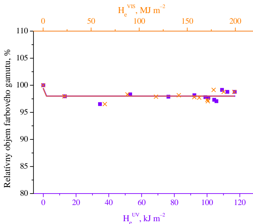
Obr. 84 Pokles relatívneho objemu farebného gamutu testovacej škály na papieri Ilford Classic Gloss, umiestnenej v ráme so sklom, v závislosti na dávke ožiarenia.
