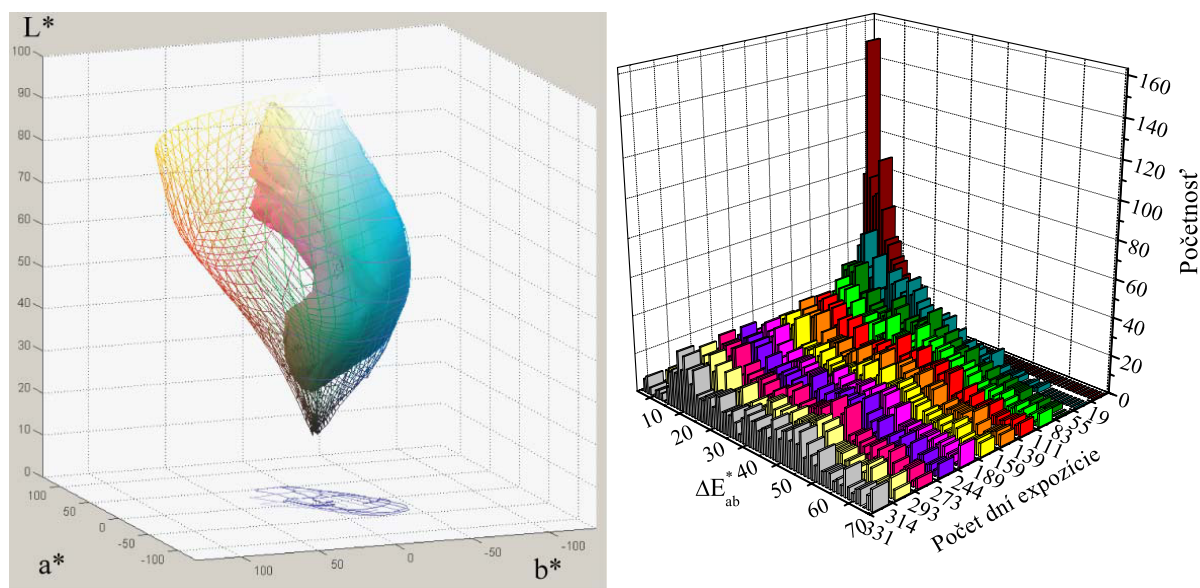
Obr. 65 Vľavo: zmena objemu farebného gamutu testovacej škály na papieri Epson Archival Matt, umiestnenej v ráme so sklom. Pred expozíciou (sieť) a po expozícii (plný objem). Vpravo: početnosť farebných odchýlok (viď Tabuľka 10).
