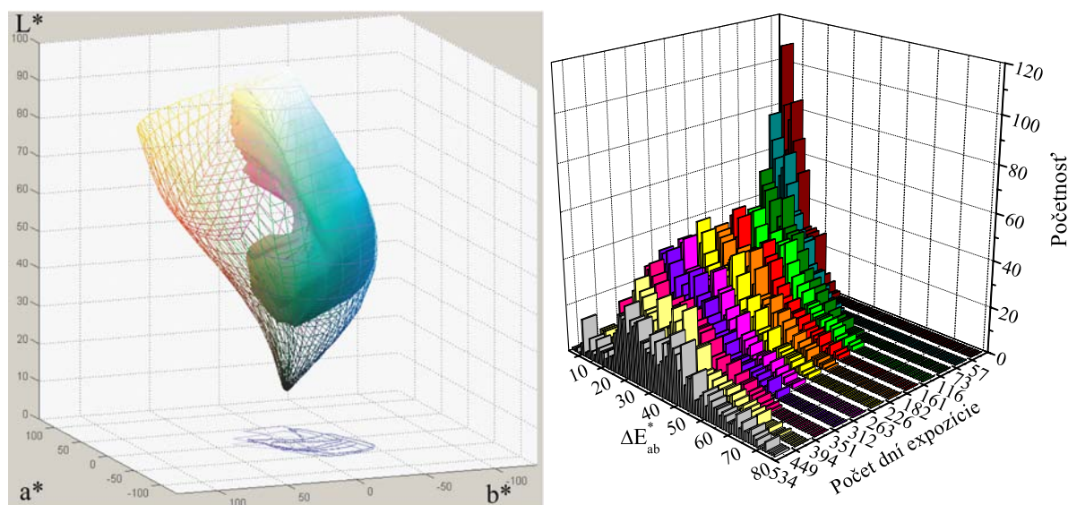
Obr. 51 Vľavo: zmena objemu farbového gamutu na papieri Foma 1224 pred expozíciou (sieť) a po 534 dňoch expozície (plný objem). Vpravo: početnosť farbových odchýlok (viď Tabuľka 7).
