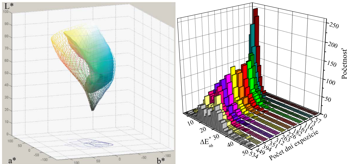
Obr. 59 Vľavo: zmena objemu farbového gamutu na papieri Chagall biely pred expozíciou (sieť) a po 534 dňoch expozície (plný objem). Vpravo: početnosť farbových odchýlok (vid' Tabuľka 8).
