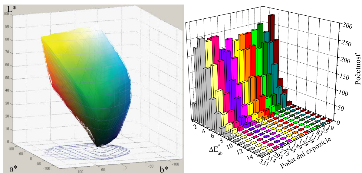
Obr. 83 Vľavo: zmena objemu farbového gamutu testovacej škály na papieri Ilford Classic Gloss, umiestnenej v ráme so sklom. Pred expozíciou (siet') a po expozícii (plný objem). Vpravo: početnosť farbových odchýlok (viď Tabuľka 12).
