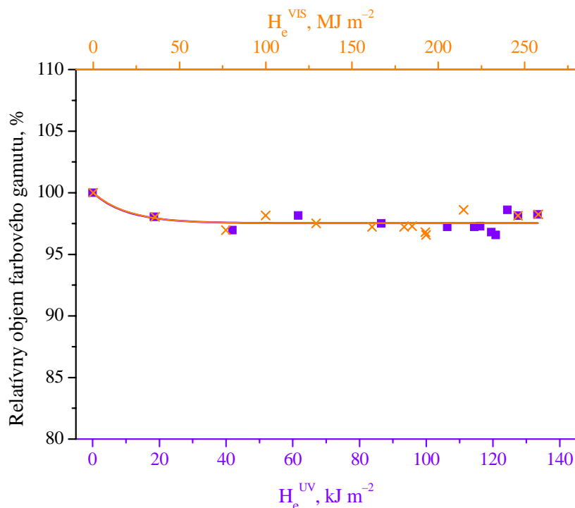
Obr. 92 Pokles relatívneho objemu farbového gamutu testovacej škály na papieri Ilford Classic Gloss, umiestnenej v ráme bez skla, v závislosti na dávke ožiarenia.
