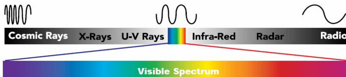
Obr. 18 Elektromagnetické spektrum. 42
