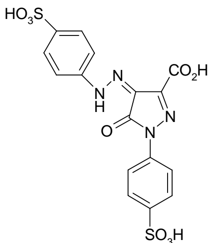
Obr. 8 Molekula žltého farbiva CI Acid Yellow 23.
