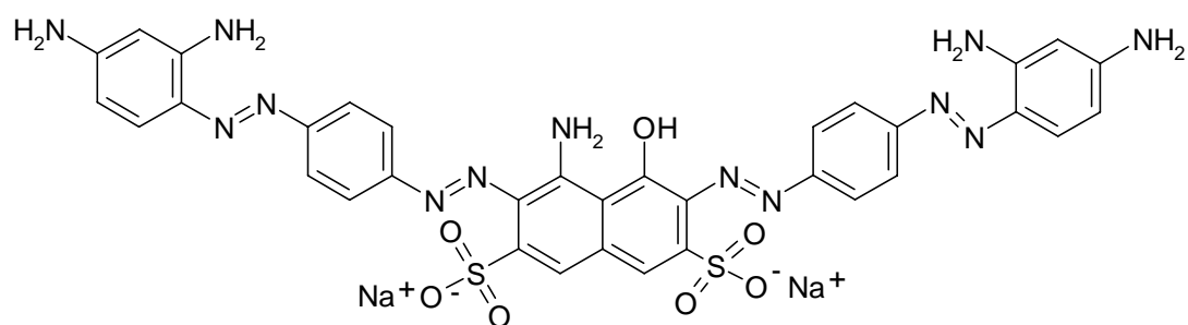
Obr. 12 Molekula čierneho farbiva CI Direct Black 19.
