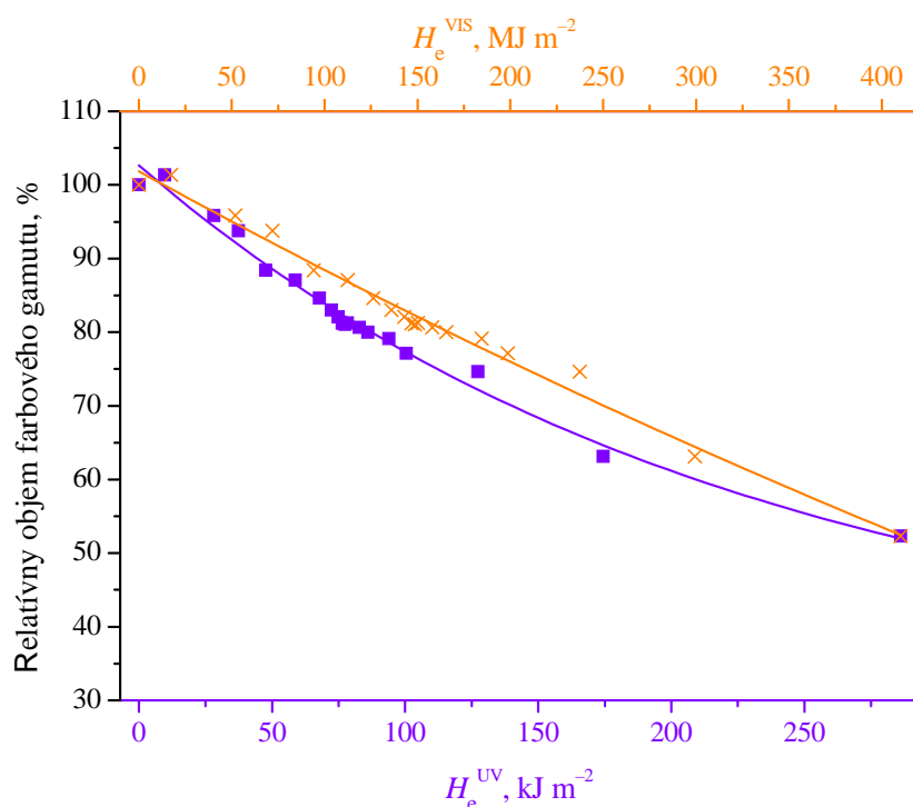
Obr. 50 Pokles relatívneho objemu farbového gamutu na papieri Epson Premium Glossy v závislosti na dávke ožiarenia.
