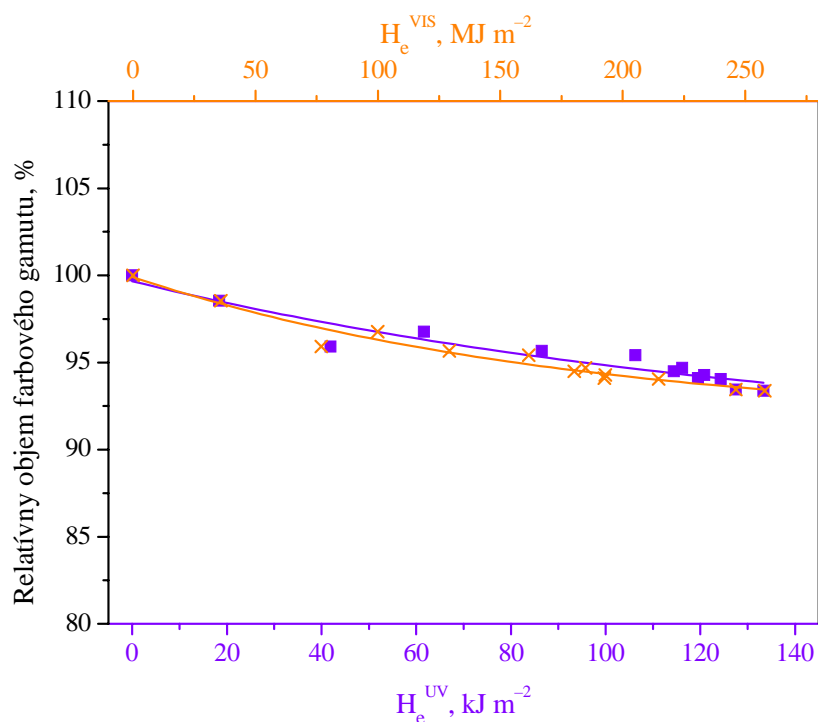
Obr. 90 Pokles relatívneho objemu farbového gamutu testovacej škály na papieri Epson Archival Matt, umiestnenej v ráme bez skla, v závislosti na dávke ožiarenia.
