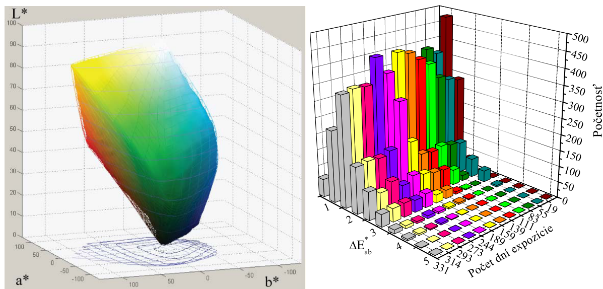
Obr. 93 Vľavo: zmena objemu farebného gamutu testovacej škály na papieri Ilford Smooth Gloss, umiestnenej v ráme bez skla. Pred expozíciou (sieť) a po expozícii (plný objem). Vpravo: početnosť farebných odchýlok (vid' Tabuľka 13).
