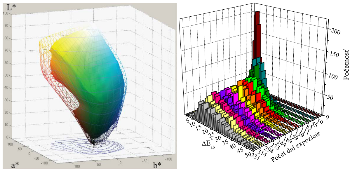
Obr. 75 Vľavo: zmena objemu farbového gamutu testovacej škály na papieri Ilford Classic Gloss, umiestnenej v ráme bez skla. Pred expozíciou (sieť) a po expozícii (plný objem). Vpravo: početnosť farbových odchýlok (viď Tabuľka 11).
