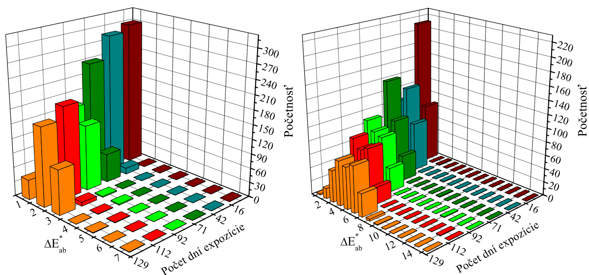
Obr. 105 Početnosť farebných odchýlok na papieri Hahnemühle Glossy Cellulose. Vľavo: umiestnený v ráme so sklom (vid' Tabuľka 17), vpravo: umiestnený v ráme bez skla (vid' Tabuľka 16).
