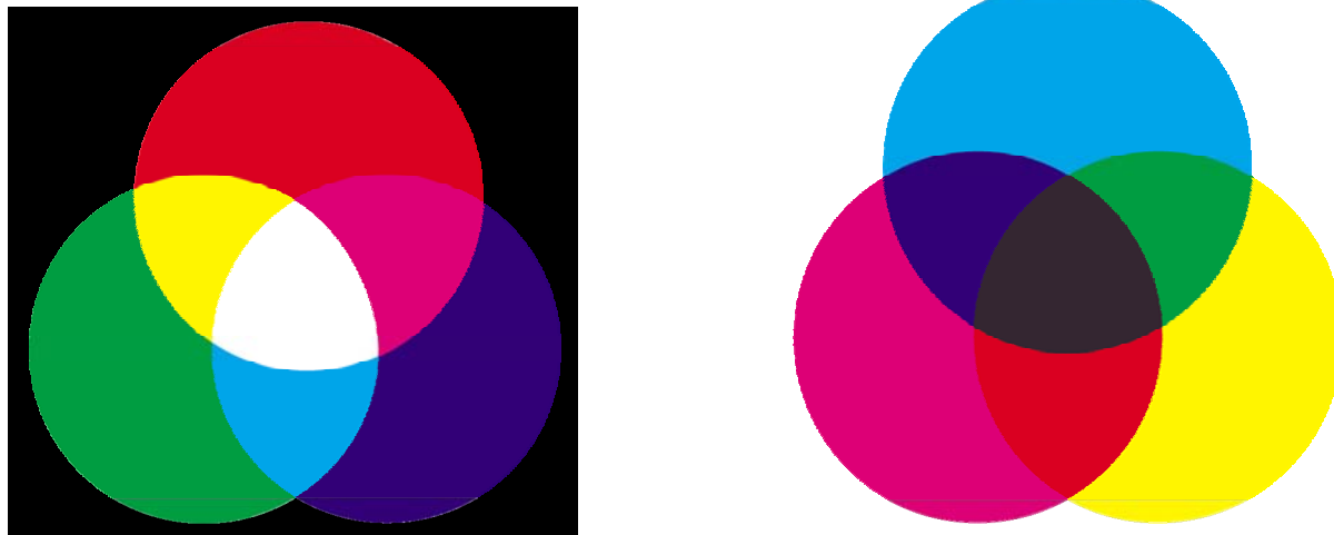
Obr. 20 Miešanie farieb: vľavo aditívne, vpravo subtraktívne. 46
