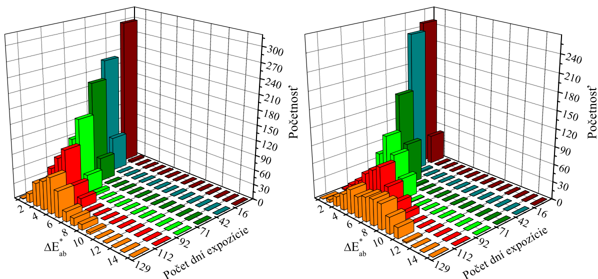
Obr. 102 Početnosť farbových odchýlok na papieri Foma 1224. Vľavo: umiestnený v ráme so sklom (vid' Tabuľka 17), vpravo: umiestnený v ráme bez skla (vid' Tabuľka 16).
