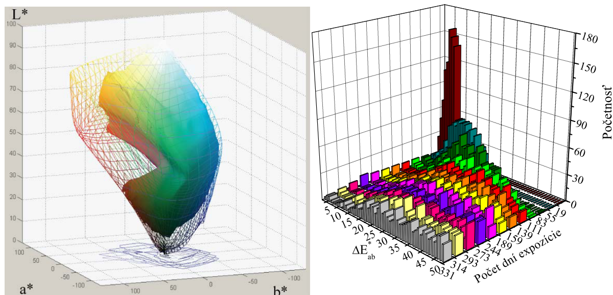
Obr. 67 Vľavo: zmena objemu farbového gamutu testovacej škály na papieri Ilford Classic Gloss, umiestnenej v ráme so sklom. Pred expozíciou (siet') a po expozícii (plný objem). Vpravo: početnosť farbových odchýlok (vid' Tabuľka 10).
