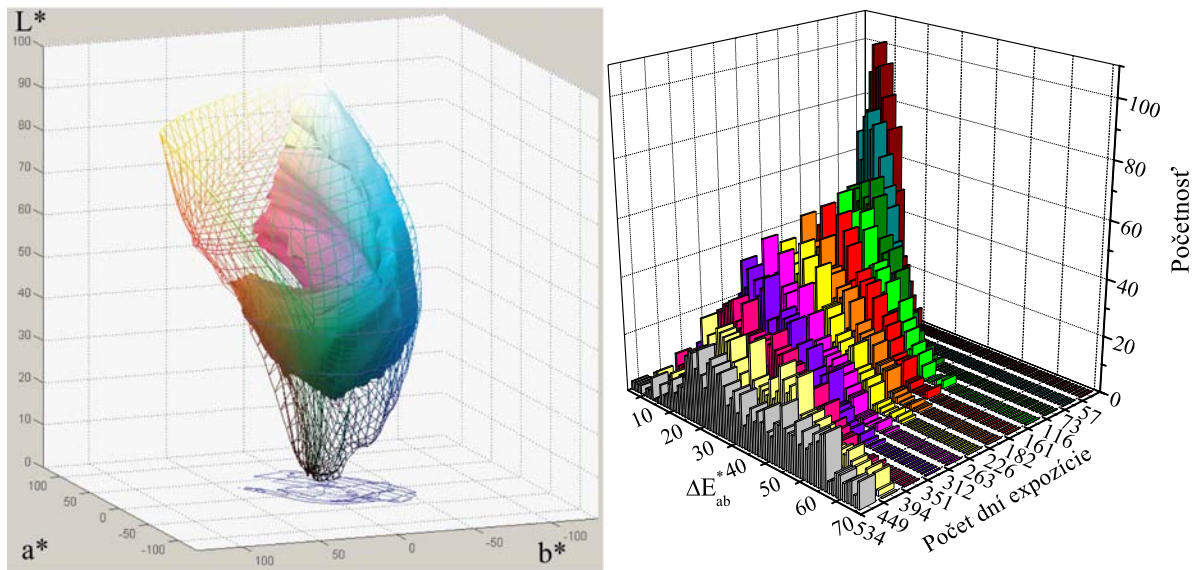
Obr. 47 Vľavo: zmena farbového gamutu na papieri Ilford Classic Gloss pred expozíciou (sieť) a po 534 dňoch expozície (plný objem). Vpravo: početnosť farbových odchýlok (viď Tabuľka 7).
